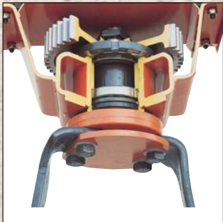
Unidad de rotor con alojamiento intercambiable
