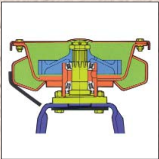
Unidad de rotor y chasis
