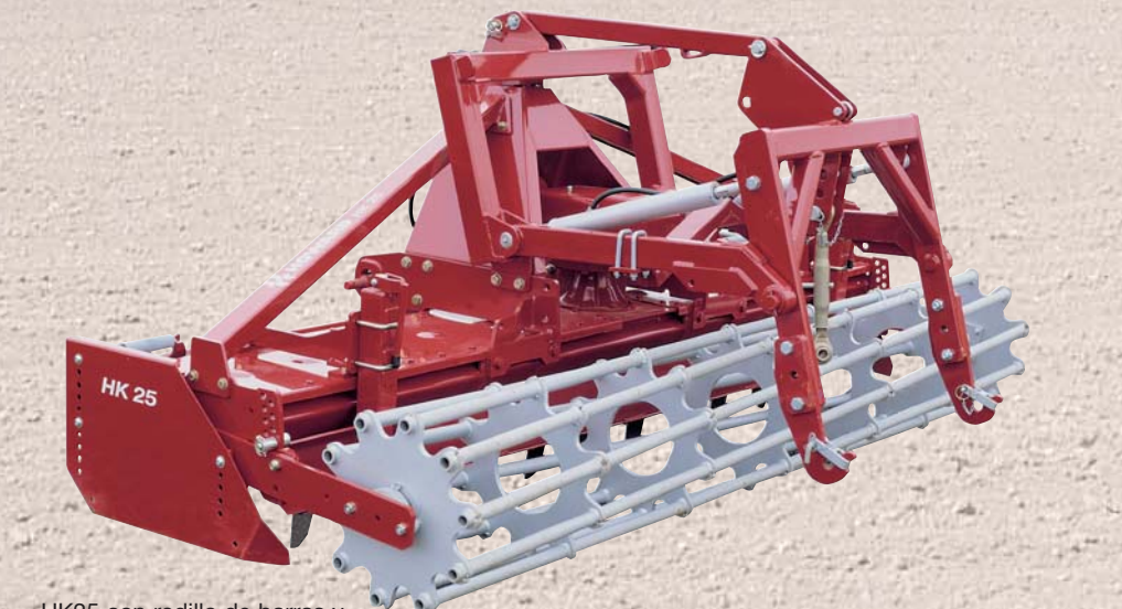
HK25 con rodillo de barras y tripuntal hidráulico opcional
