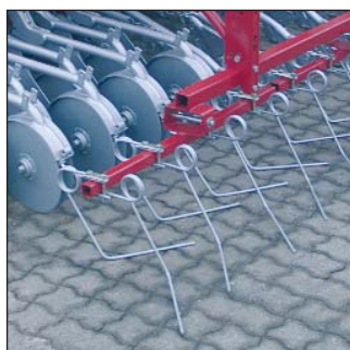
Rastrillo opcional Wing-Flow.
