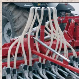
Los tubos de igual longitud permiten una dosificación igual en todas las salidas.
