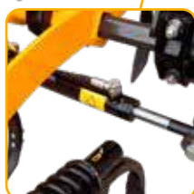
Martinetti idraulici per apertura telaio Hydraulic jacks for opening frame Vérins hydrauliques pour l'ouverture du châssis Hydraulikzylinder zum Öffnen des Rahmens
