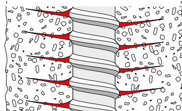
Aperturas de fisura s < 0,1 \text{ mm} comprobadas en estado de agotamiento del acero
