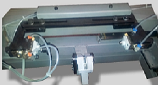
Mecanismo de cajeadó para cerraduras.
