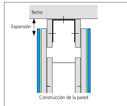
JUNTA DESLIZANTE: TECHO
