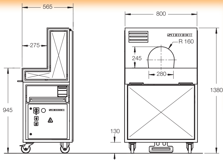
Dimensiones de la máquina y el túnel
