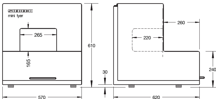
Dimensiones de la Máquina
