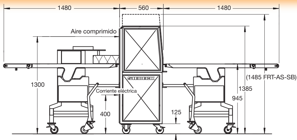
Dimensiones de la máquina
