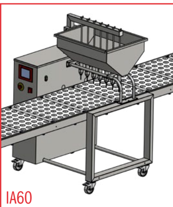
Dosificador de azúcar glass
