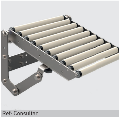
Rampa de salida de A200 mm
