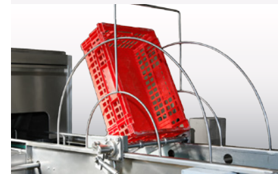
líneas de lavado de cajas y bandejas washing lines of crates and trays
