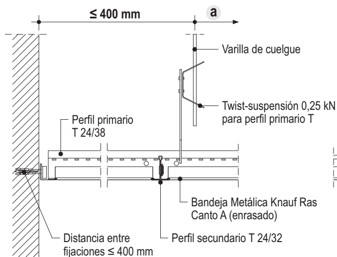
D427a-A5 Banda perimetral con angular transversal al perfil primario
