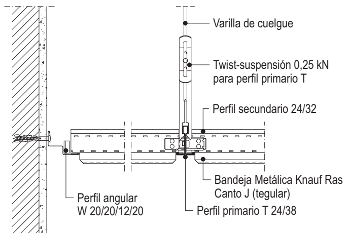
D427q-A4 Encuentro entre primario y secundario
