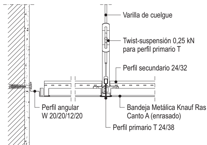
D427a-A4 Encuentro entre primario y secundario
