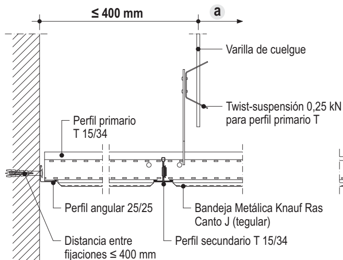
D427q-A5 Banda perimetral con angular transversal al perfil primario
