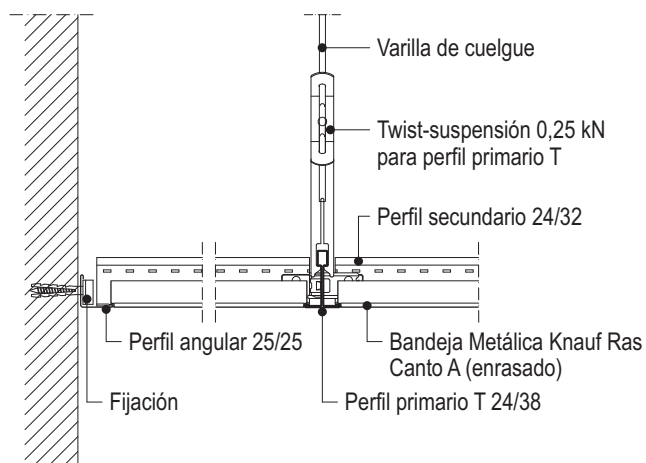
D427a-A3 Banda perimetral con angular transversal al perfil primario
