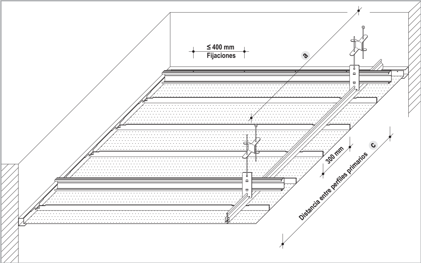
Separación entre perfiles
