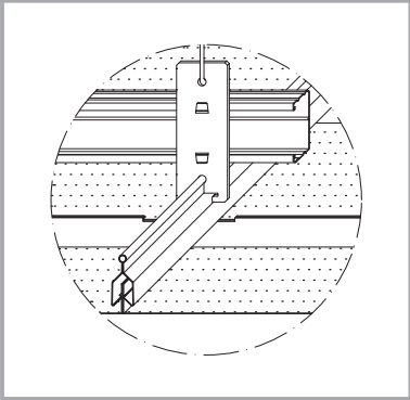
Encuentro con bandeja y perfiles
