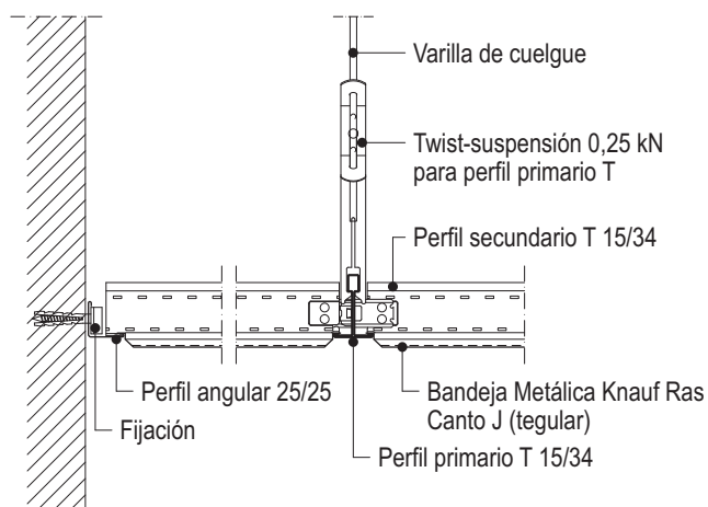
D427q-A3 Banda perimetral con angular transversal al perfil primario
