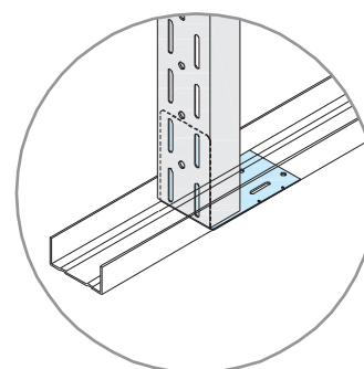
Anclaje inferior
