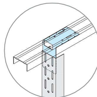
Anclaje superior
