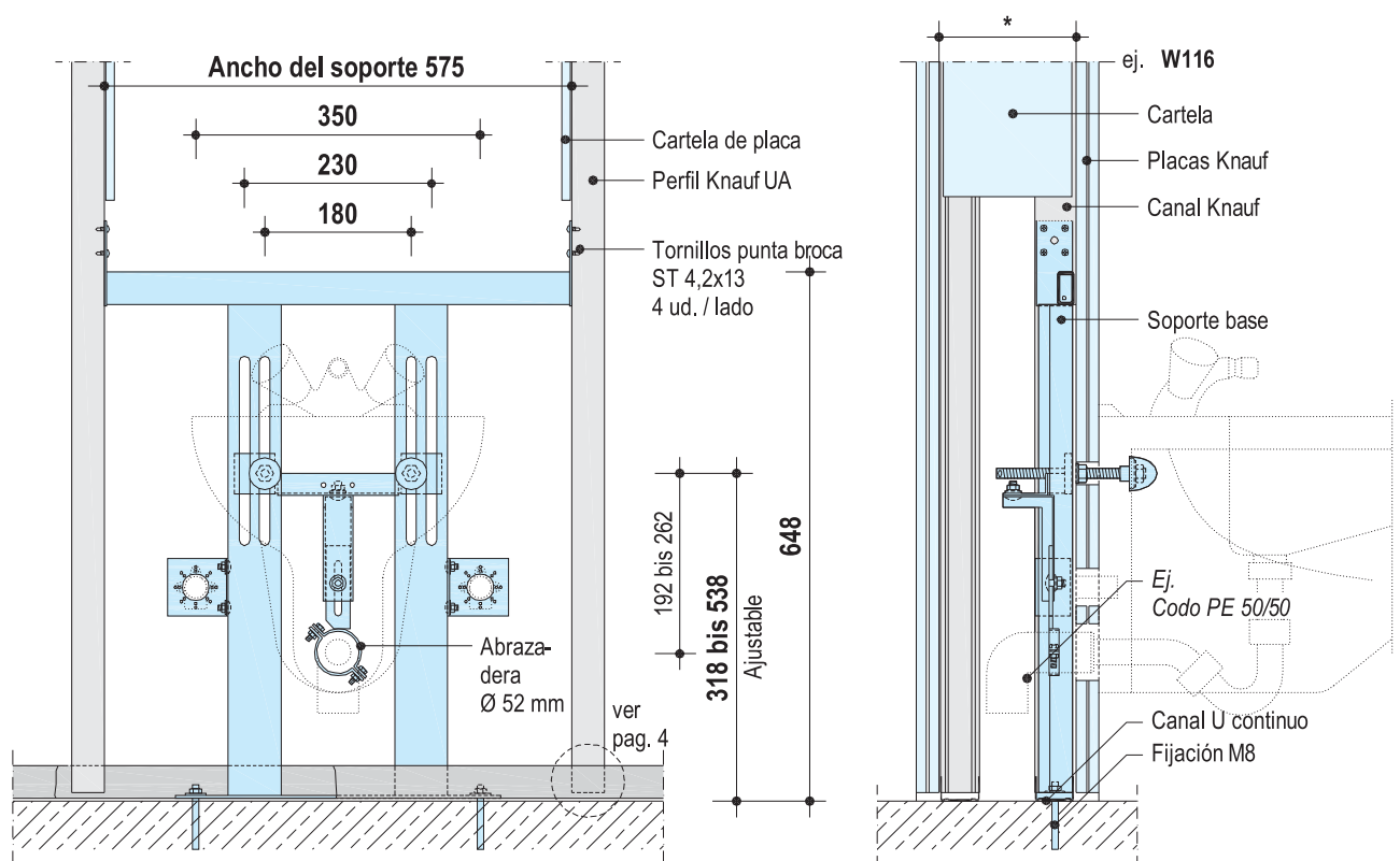
W223-A12 Vista frontal
