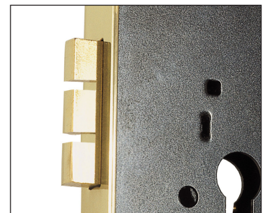
Palancas anticorte y antitaladro.
