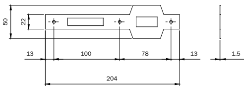
Cerradero plano, bordes cuadrados, con doble aleta para serie: 280N. ACERO LATONADO 204x22x1,5 mm
