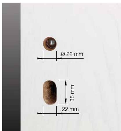
Preparación de la puerta interior: para manillas con Mini-Roseta, con bocallave
