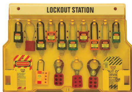
ESTACIÓN ALMACENAJE B 20 CANDADOS LOCKOUT STATION B 20 PADLOCKS
