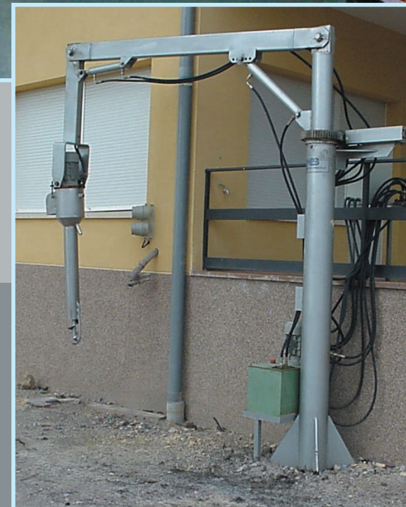
PINCHOS TOMAMUESTRAS
