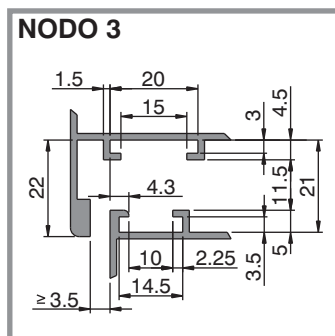
PLATINA DOBLE Y ANTI-ELEVACIÓN
