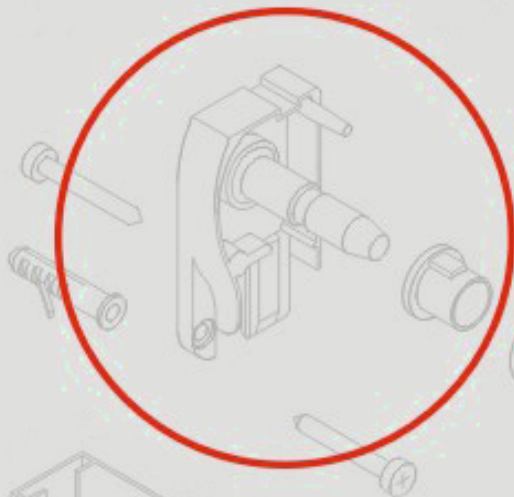
Testero con tornillo de sujeción al cajón. Fastening of end cap at the box.
