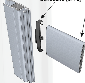
Pieza Sujeción travesaño (1772)
