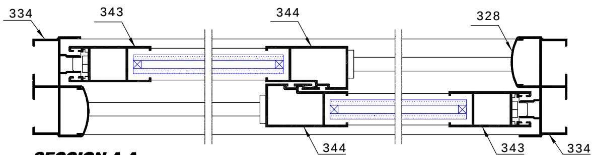
SECCION A-A
