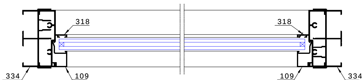
SECCION B-B
