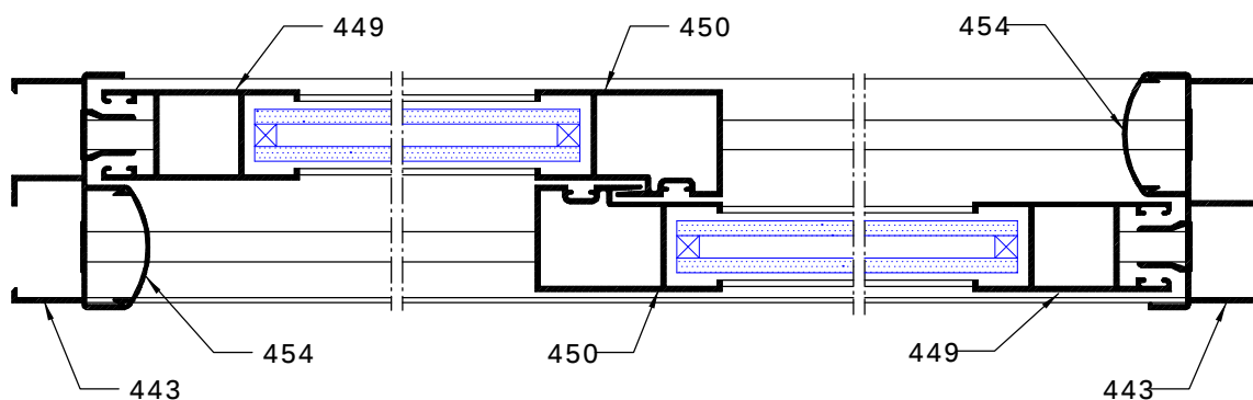
SECCION A-A
