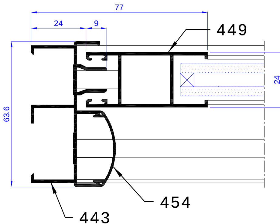
Nudo lateral corredera
