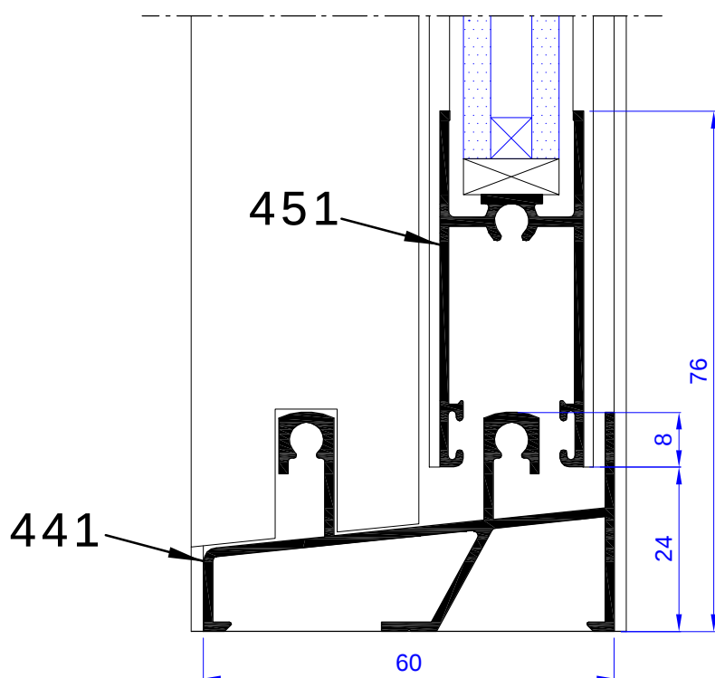
Nudo inferior corredera
