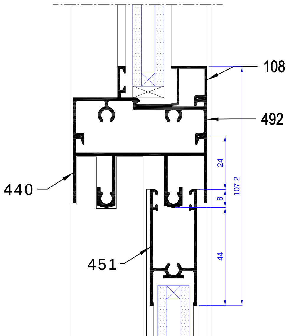
Nudo central montante superior
