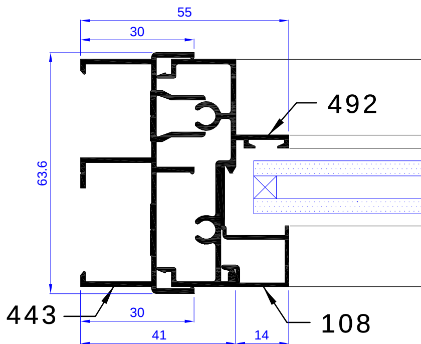
Nudo lateral fijo
