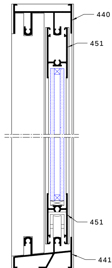
SECCION B-B
