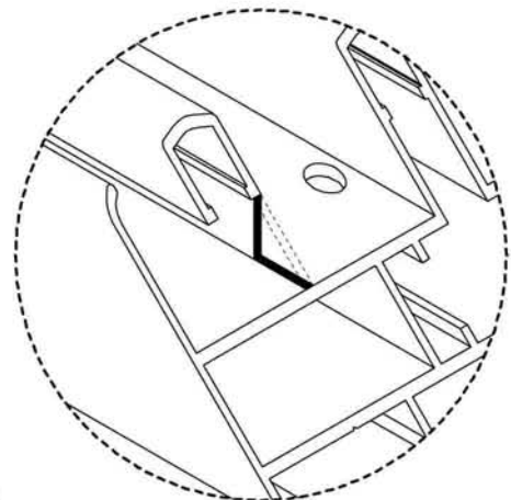
DETALLE 1
