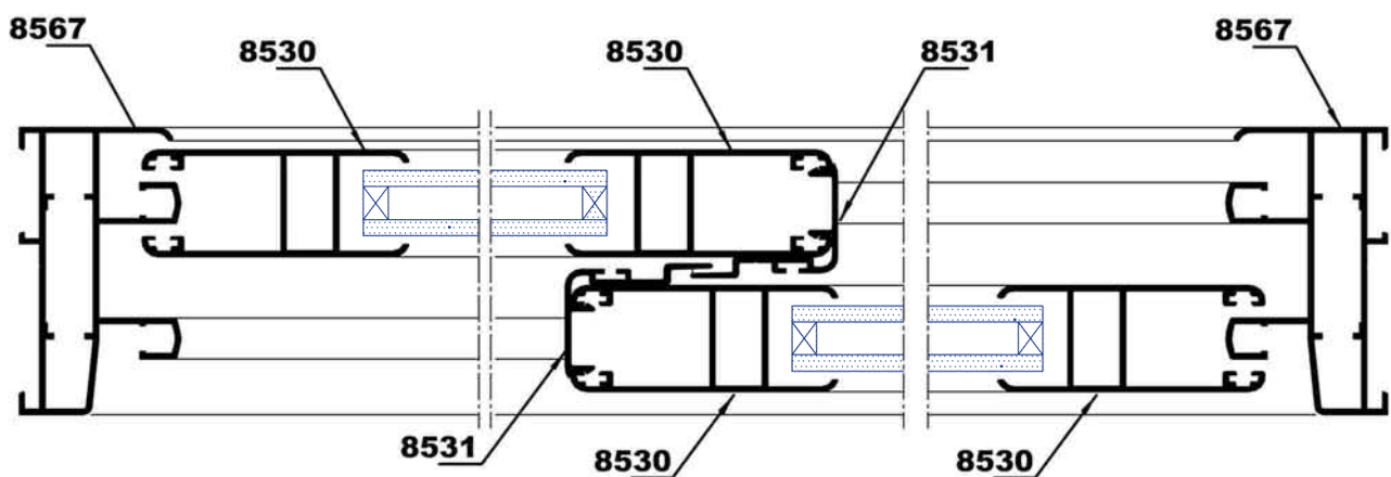
SECCION A-A
