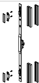
4187 Cierre multipunto H: 668-1068
