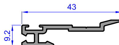
Accesorio 4111 (Barra 3 m.)
