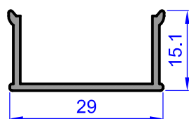
Accesorio 4110 (Barra 3 m.)
