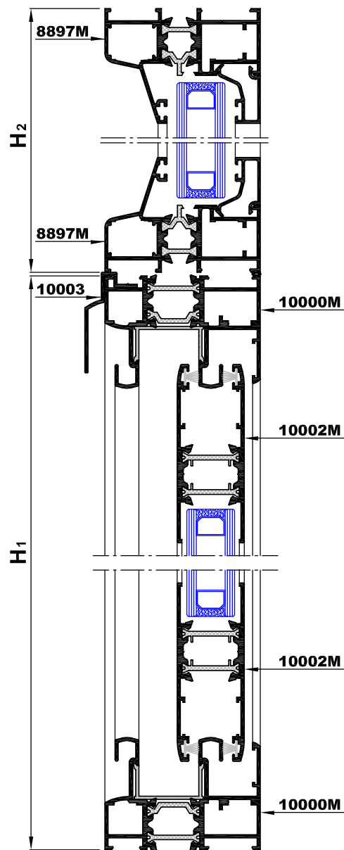
Seccion B-B
