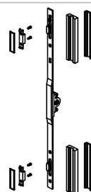
4189 Cierre multipunto H: > 1869
