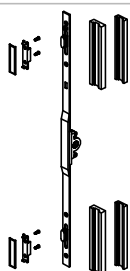
4188 Cierre multipunto H: 1069-1868
