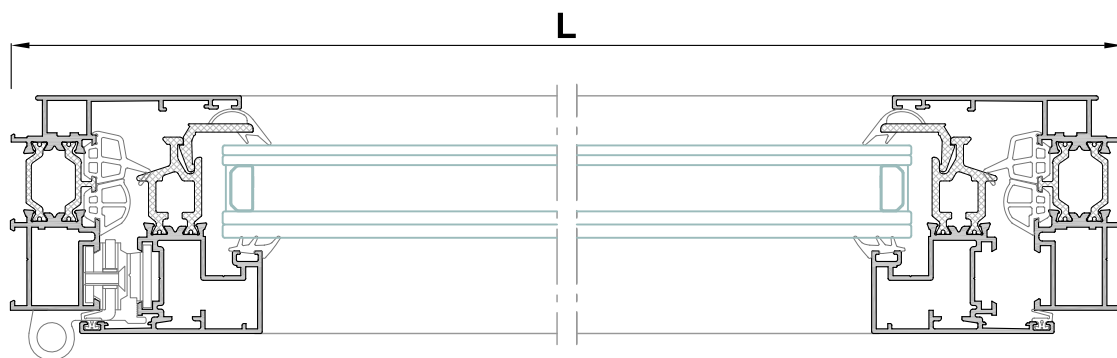
Sección A-A'
