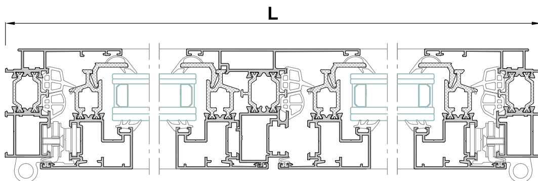
Sección A-A'
