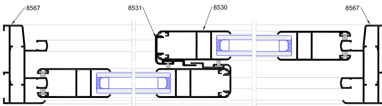
Seccion A-A'
