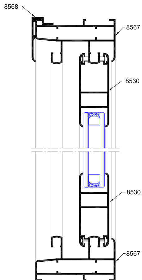
Seccion B-B'
