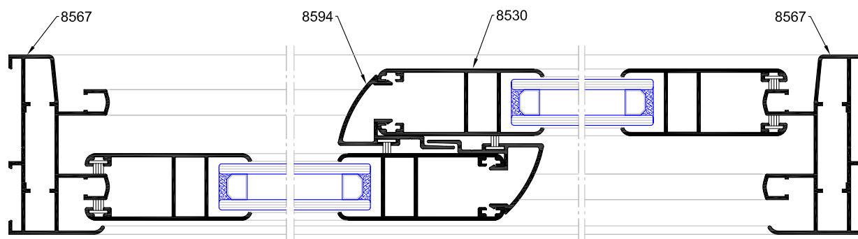
Seccion A-A'
