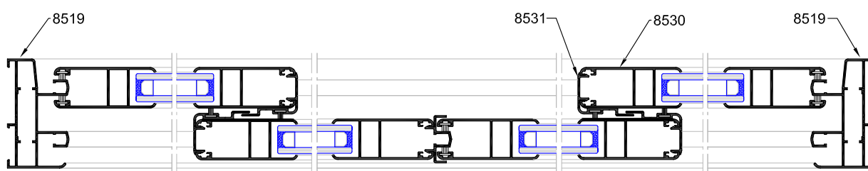
Seccion A-A'
