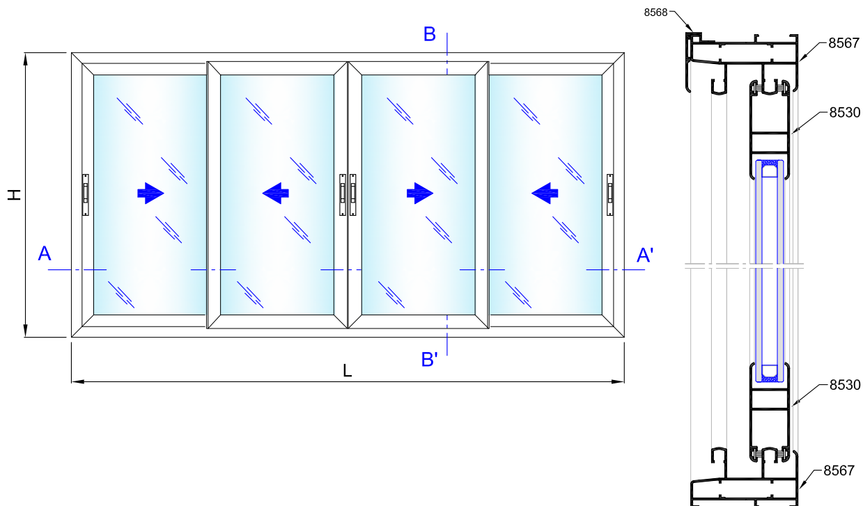
Seccion B-B'
