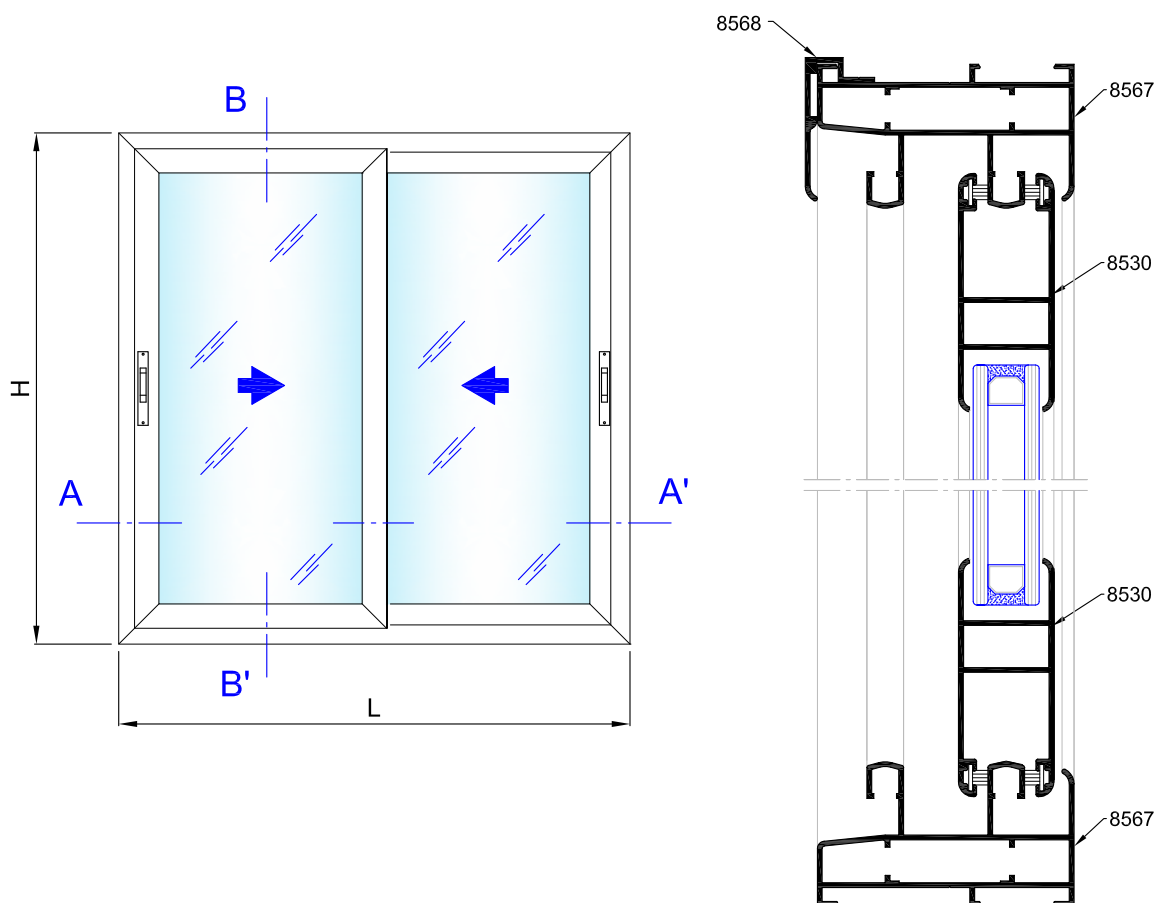
Seccion B-B'
