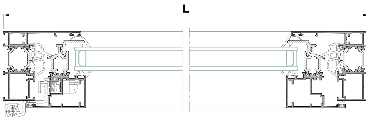
Sección A-A'
