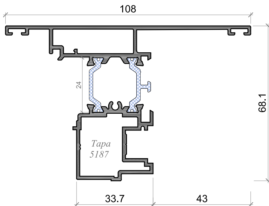
16781L | Acople Inversora alg 65 HS C16
