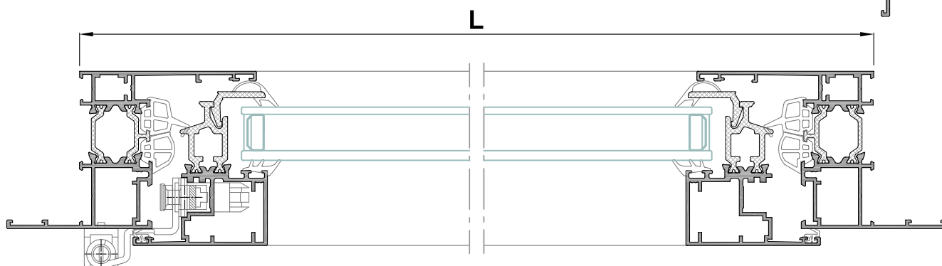
Sección A-A'
