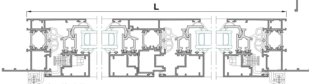
Sección A-A'
