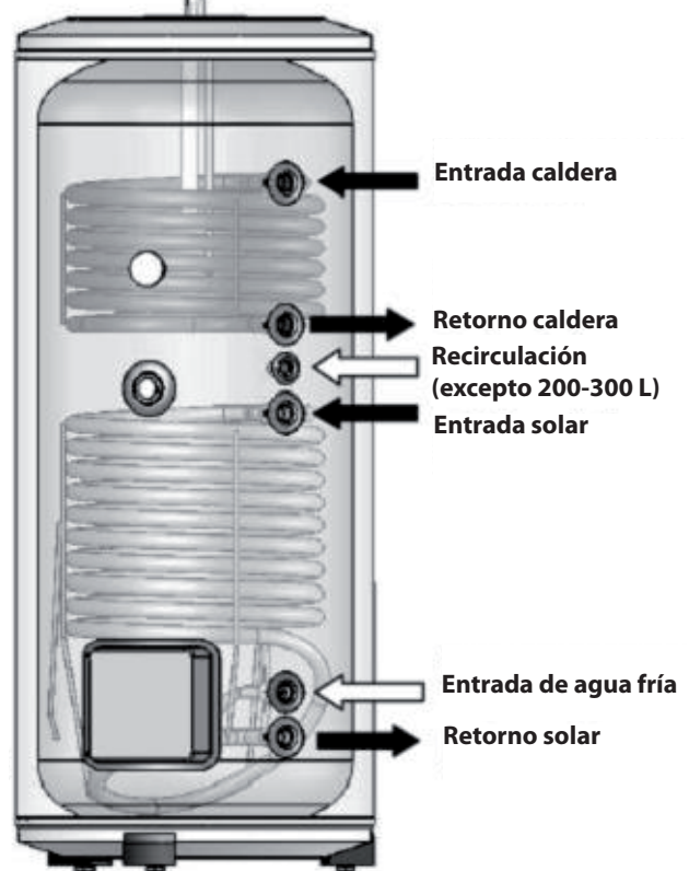
ACUMULADOR 2S ↑ Salida de agua caliente
