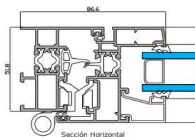
Sección Horizontal
