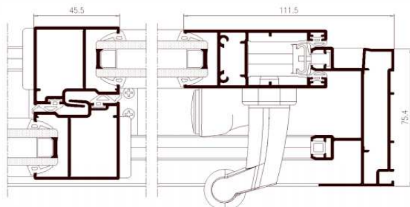
SIN ROTURA
