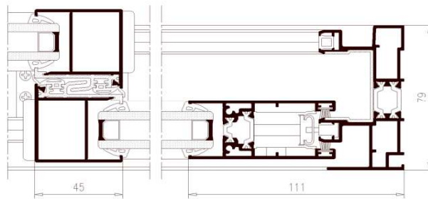
CON ROTURA
