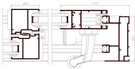
SIN ROTURA
