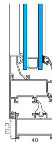
Sección Vertical
