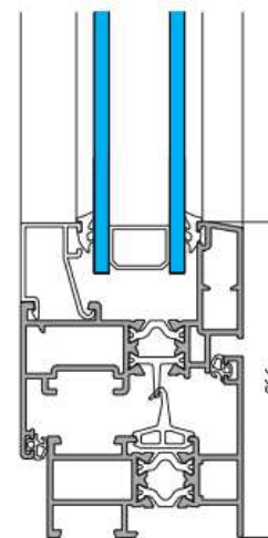
Sección Vertical
