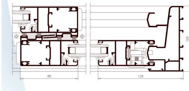
Sección
