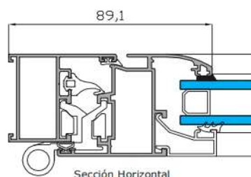
Sección Horizontal
