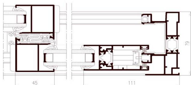
CON ROTURA
