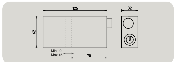
Ejemplo de instalación de Toy TC-3
