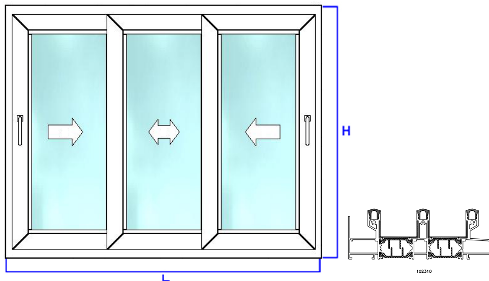
2 KITS CORREDERA HERMET - II / 3 HOJAS 3 CARRILES
