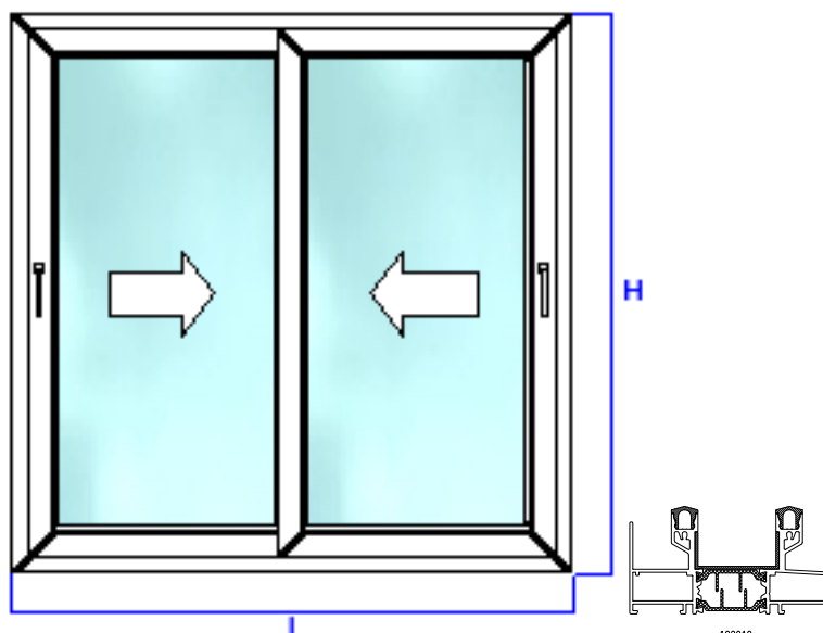
KIT CORREDERA HERMET - 1 / 2 HOJAS
