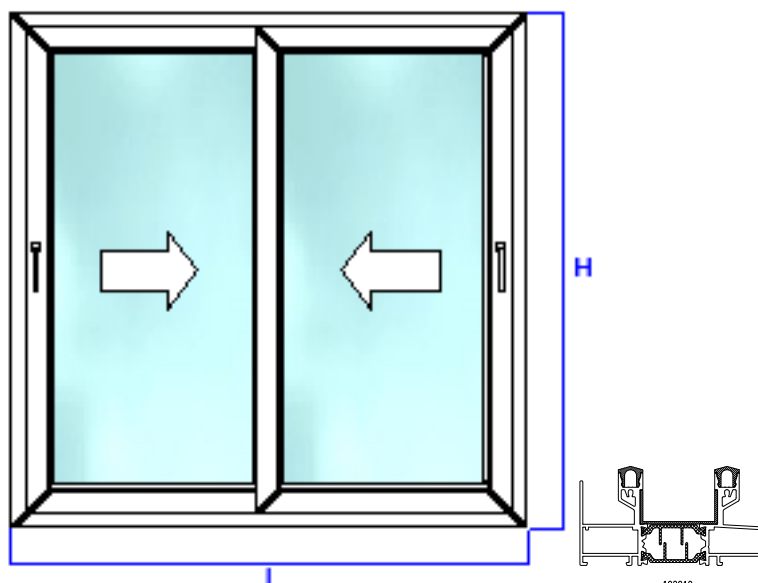
KIT CORREDERA HERMET - II / 2 HOJAS
