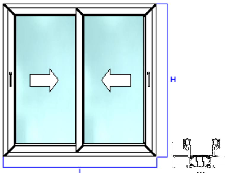
KIT CORREDERA HERMET-II ESPECIAL / 2 HOJAS 2 CARRILES
