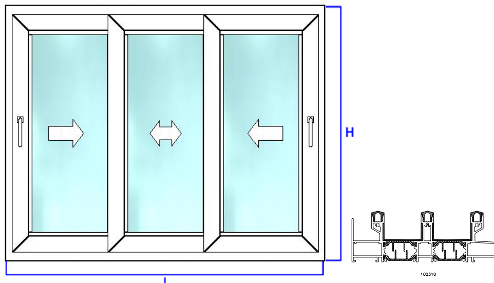
KIT CORREDERA HERMET - I / 3 HOJAS 3 CARRILES
