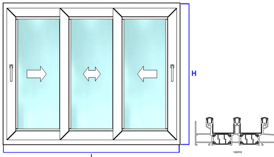
2 KITS CORREDERA HERMET - III / 3 HOJAS 3 CARRILES
