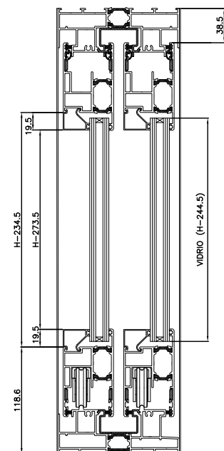
SECCION B-B'
