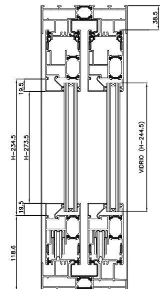
SECCION B-B'
