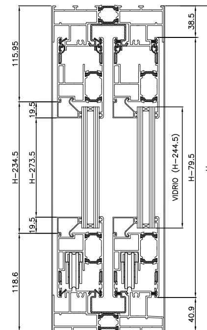
SECCION B-B'
