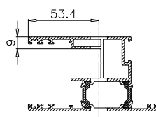
MECANIZADO MANILLA
