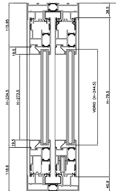
SECCION B-B'
