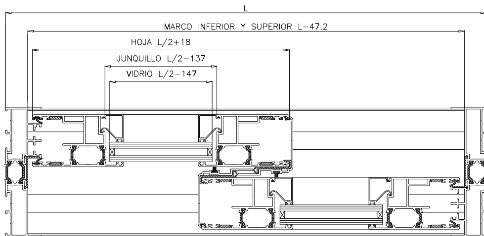
SECCION A-A'
