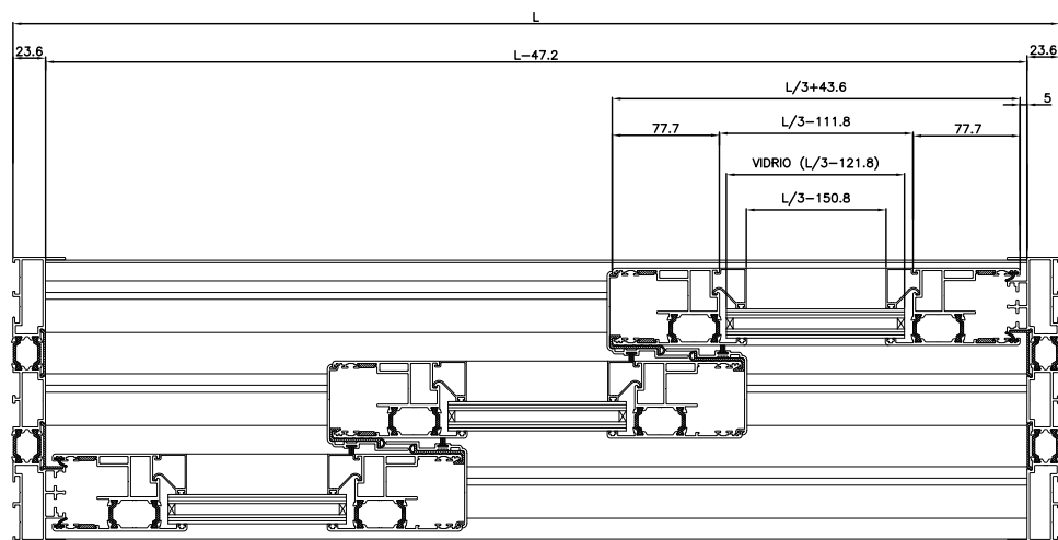
SECCION A-A'
