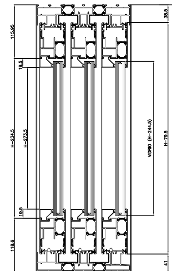
SECCION B-B'
