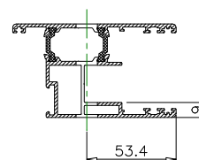
MECANIZADO MANILLA
