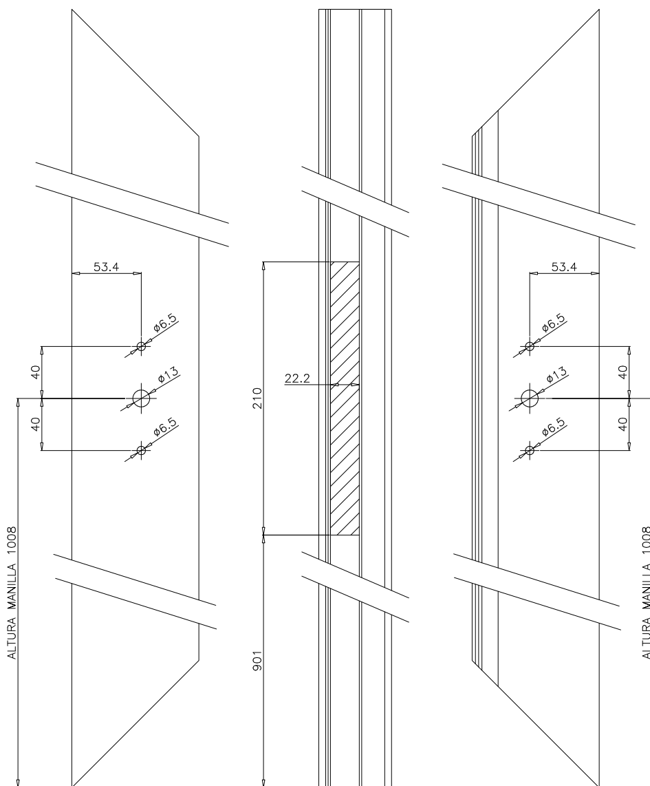
MECANIZADO MANILLA
