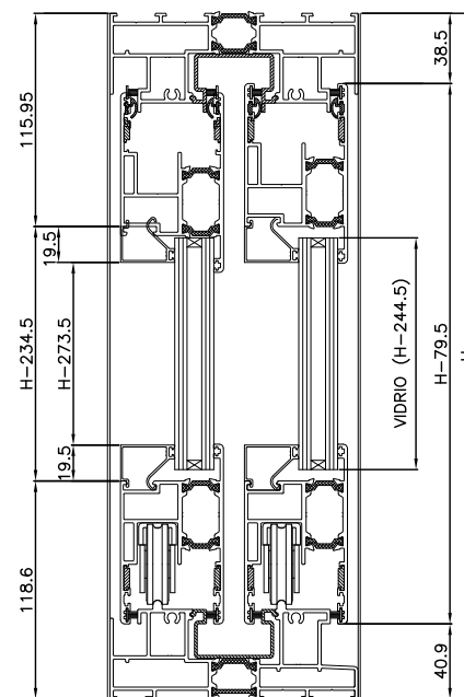
SECCION B-B'
