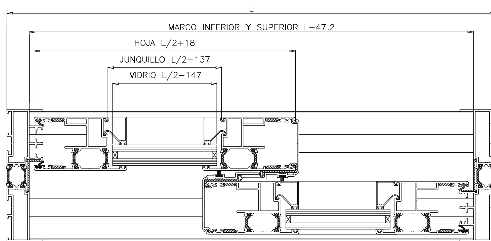
SECCION A-A'
