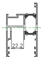
MECANIZADO CREMONA
