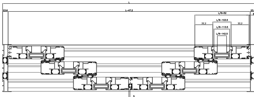
SECCION A-A'
