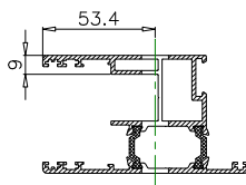
MECANIZADO MANILLA
