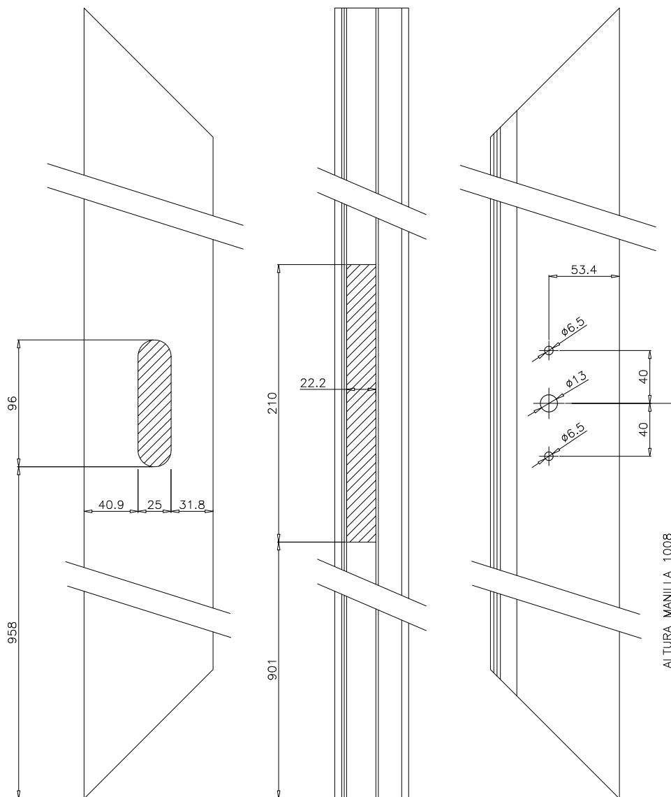
MECANIZADO UÑERO
