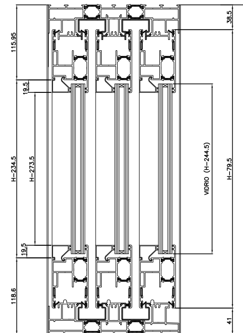
SECCION B-B'
