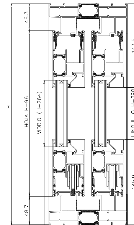
SECCION B-B'
