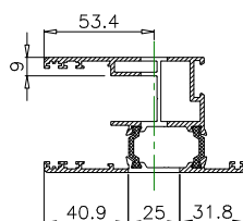
MECANIZADO UÑERO
