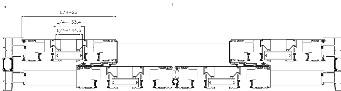
SECCION A-A'
