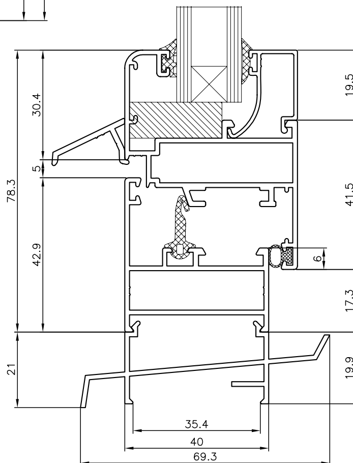
NUDO INFERIOR VENTANA CON PERFIL RECOGECONDENSACIONES
