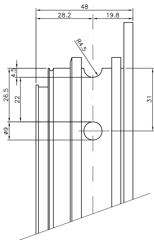
ESCUADRA (ref. 94.92.01)
