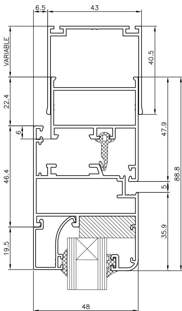
NUDO SUPERIOR CON COMPENSADOR
