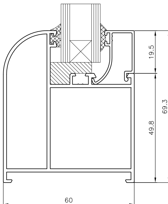
MARCO FIJO ESCAPARATE MARCO 943614
