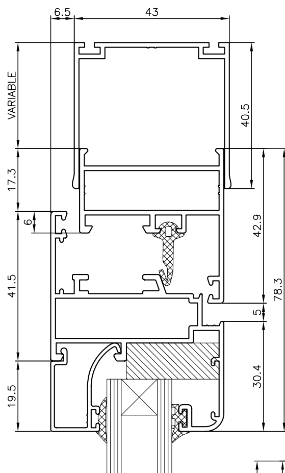
NUDO SUPERIOR CON COMPENSADOR
