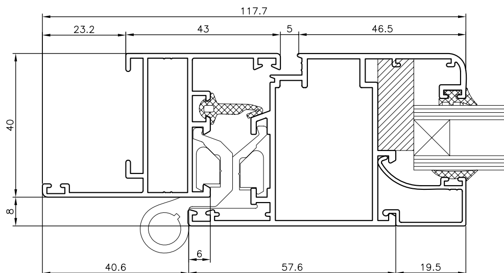
NUDO LATERAL PERFIL BALCONERA 942720 Y MARCO 941111
