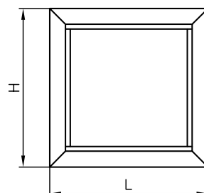
MARCO 941614
