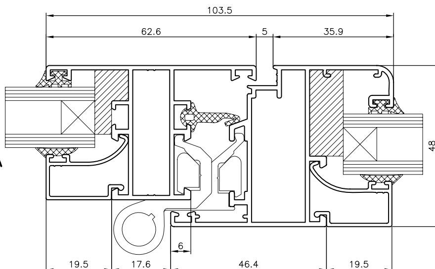
LATERAL FIJO Y PERFIL VENTANA APERTURA INTERNA MARCO 941130 HOJA 941620
