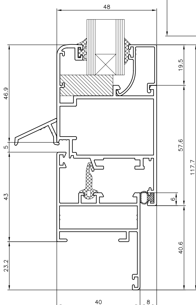
NUDO INFERIOR PERFIL BALCONERA MARCO CON SOLAPE MARCO 941111 HOJA 942720
