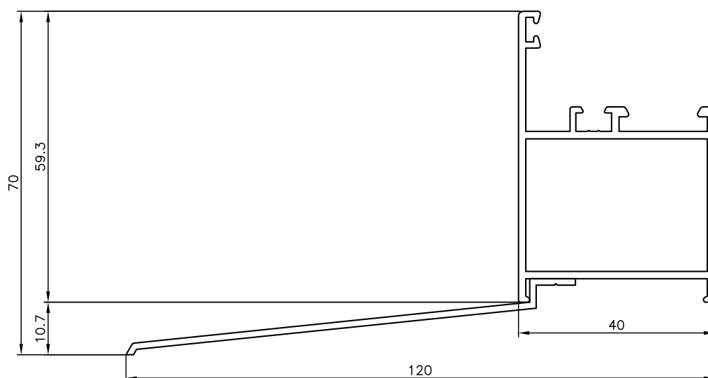
MARCO 942710 Y VIERTEAGUAS 4657
