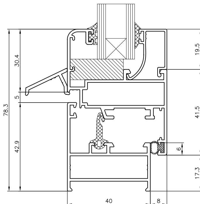
NUDO INFERIOR VENTANA MARCO 941110 Y HOJA 941120
