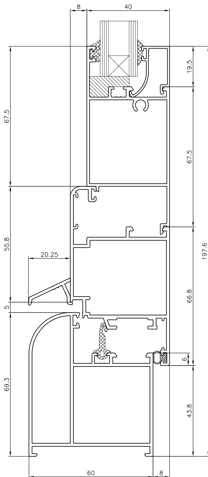
NUDO INFERIOR PERFIL PUERTA CON SUPLEMENTO ZOCALO MARCO 943614, HOJA 943620 Y SUPLEMENTO 940415
