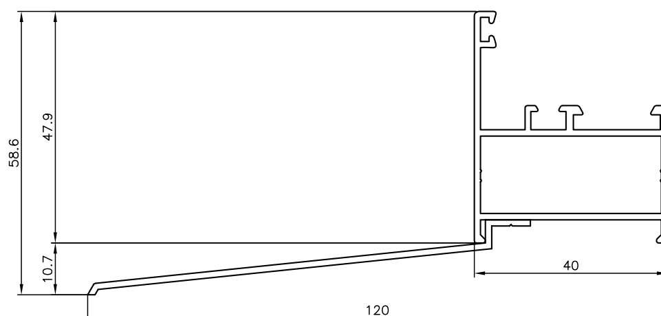
MARCO 941610 Y VIERTEAGUAS 4657
