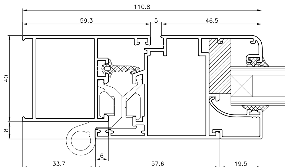
NUDO LATERAL PERFILES BALCONERA 942710 Y 942720
