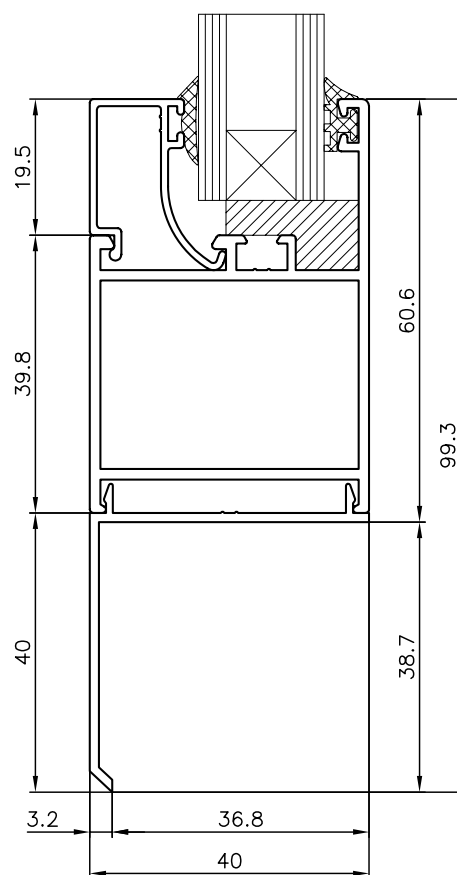
MARCO 942710 CON SOLAPE 940106
