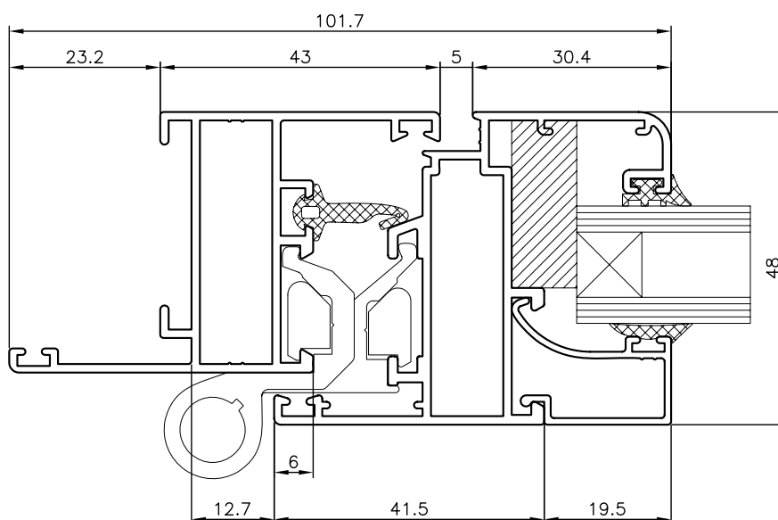
NUDO LATERAL PERFIL VENTANA MARCO CON SOLAPE MARCO 941111 HOJA 941120
