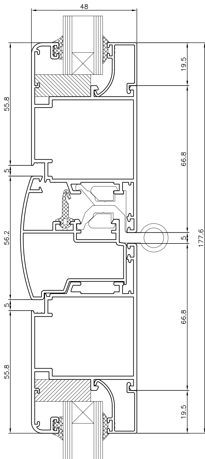
TERCERA HOJA—PUERTA APERTURA INTERNA
