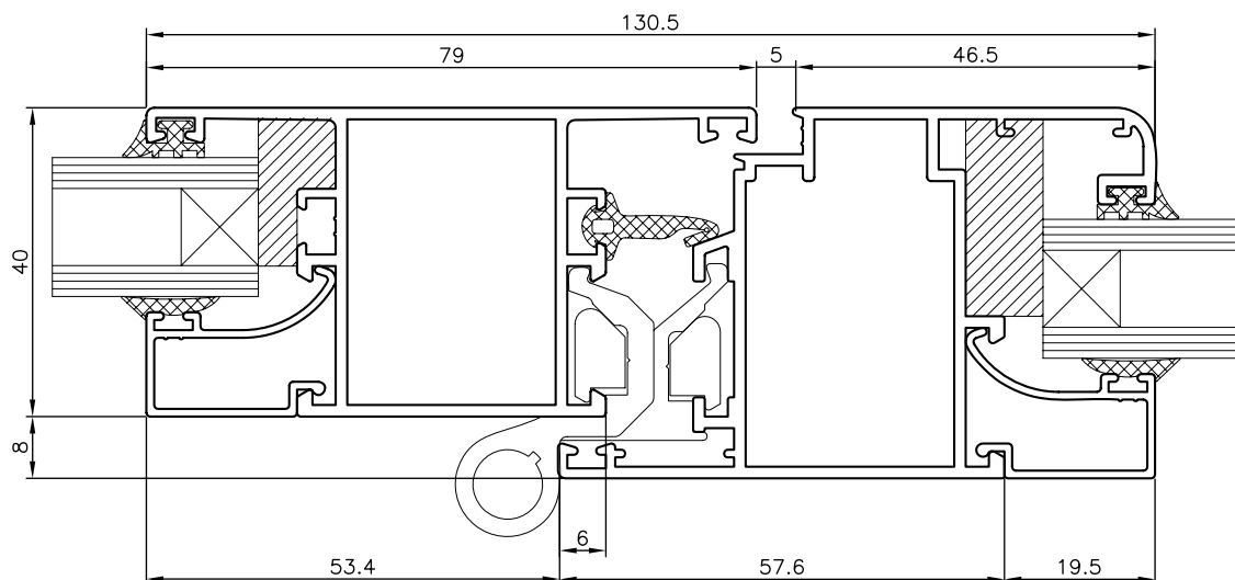
LATERAL FIJO Y PERFIL DE BALCONERA DE APERTURA INTERNA
