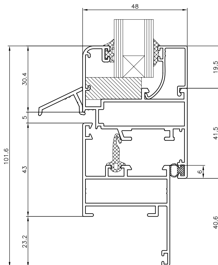
NUDO INFERIOR VENTANA MARCO CON SOLAPE MARCO 941111 Y HOJA 941120
