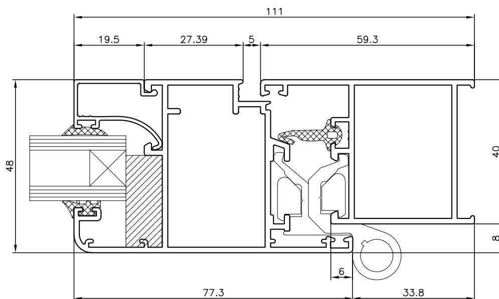
NUDO LATERAL PERFIL BALCONERA APERTURA EXTERIOR MARCO 942710 Y HOJA 942723
