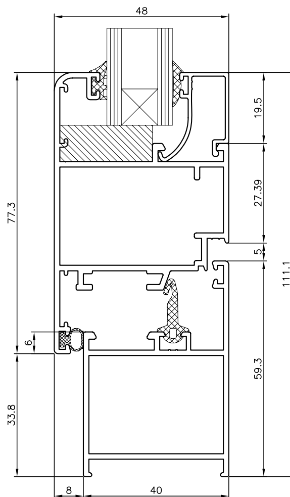
NUDO INFERIOR PERFIL BALCONERA APERTURA EXTERIOR MARCO 942710 Y HOJA 942723
