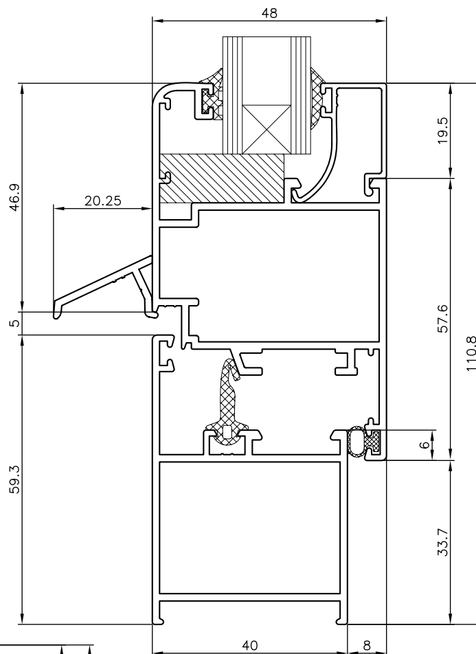
NUDO INFERIOR PERFIL BALCONERA MARCO 942710 HOJA 942720
