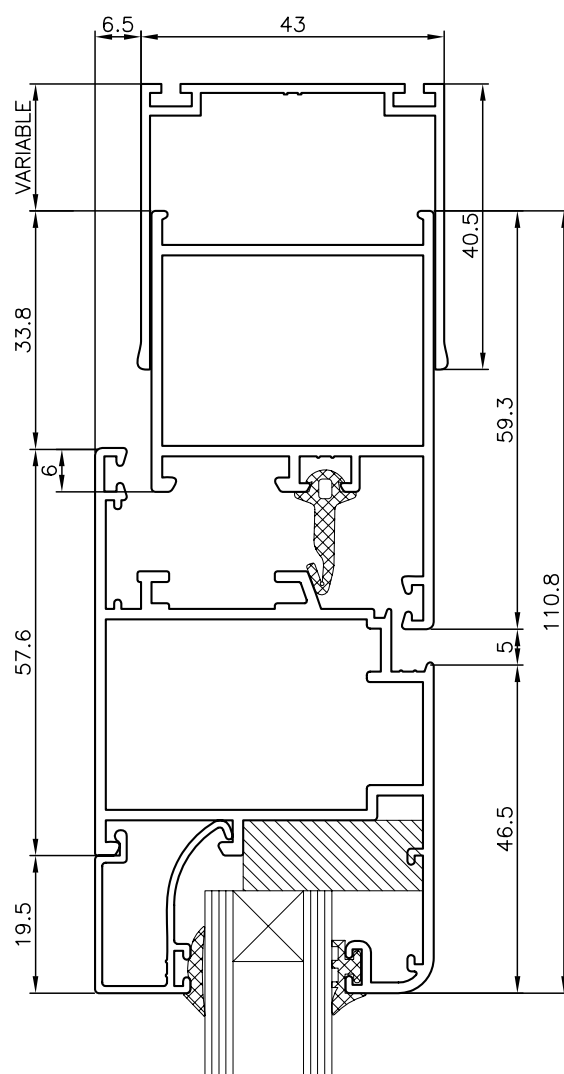
NUDO SUPERIOR CON COMPENSADOR
