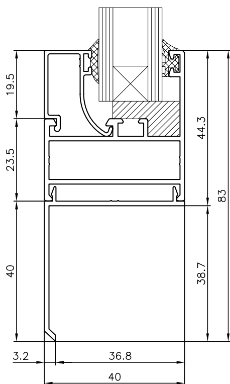
MARCO 941110 CON SOLAPE 940106
