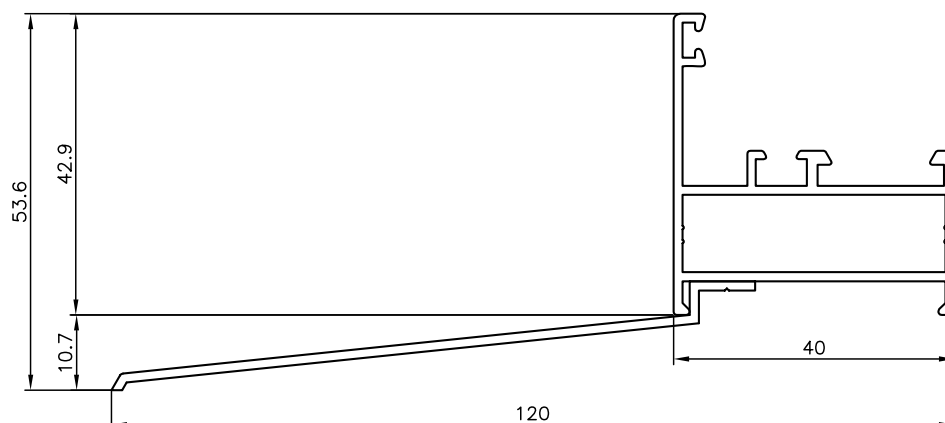
MARCO 941110 Y VIERTEAGUAS 4657
