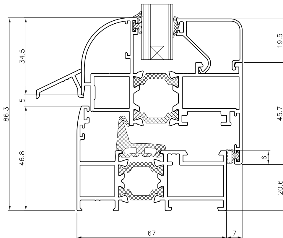
NUDO INFERIOR VENTANA MARCO 9801410 Y HOJA 9801420
