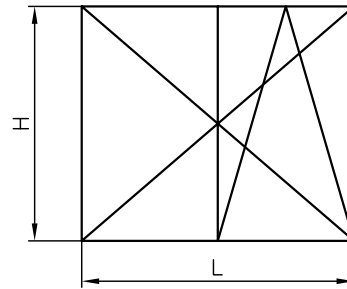
MARCO 9801410 - HOJA 9801420
