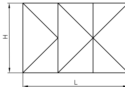
MARCO 9803210 - HOJA 9803220
