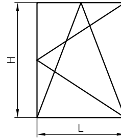
MARCO 9801410 - HOJA 9801420
