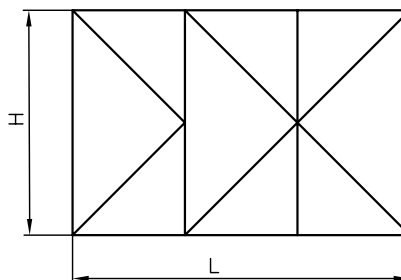
MARCO 9801410 - HOJA 9801420
