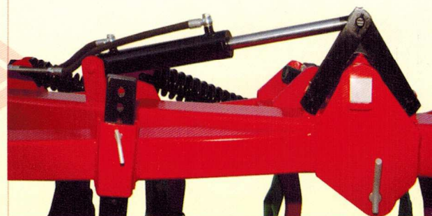
Detalle del plegado hidráulico.
