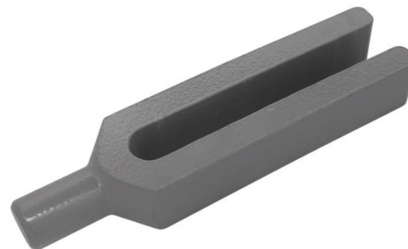
BRIDA CON EXTREMO REDONDO DIN 6315 C
