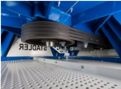
Accionamiento por correa con rodillo tensor
