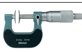
PLATILLOS
