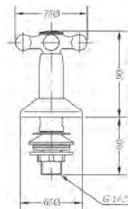
Ref.: 68520 09 45 66 Grifo bidé Bidet tap
