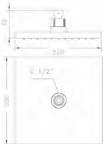
Ref.: R63112 26 Rociador cuadrado 22 cm Square shower head 22 cm Box: 1 | Carton: 24 | Pallet: 144
