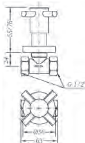
Ref.: 68170 08 45 66 Llave de paso 1/2\"/> Stopcock 1/2"
