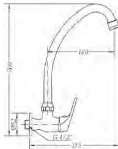
Ref.: 1005 04 Grifo mural con tubo alto 1 agua cartucho 25 One-water wall sink tap high spout 25 cartridge
