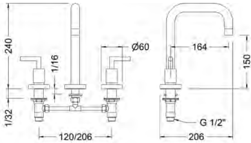
Ref.: 68120 07 45 66 Batería de lavabo caño recto Widespread wash-basin mixer with straight pipe spout
