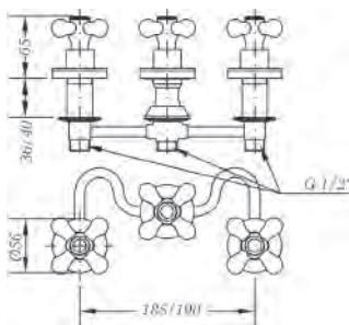
Ref.: 68142 09 45 66 Batería de bidé con transmisión Widespread bidet mixed with transmission
