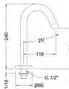
Ref.: 68917 45 Caño encimera inclinado tubo Sloping pipe spout
