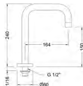
Ref.: 68915 45 Caño encimera recto tubo Straight pipe spout
