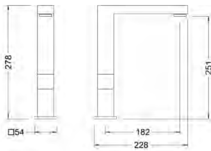
Ref.: 65208 18 60 66 Monomando de fregadera inox con cartucho progresivo Stainless steel sink mixer with progressive cartridge Box: 1 | Carton: 4
