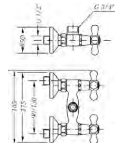
Ref.: 568550 45 Cuerpo grupo mural 11 cm Wall body mixer 11 cm
