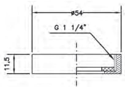
Ref.: 100134 07 Tuerca para sifon 1 1/4" 1 1/4" siphon nut
