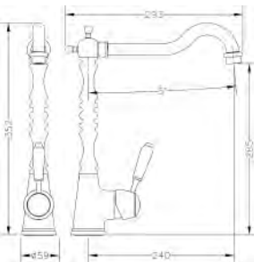
Ref.: 68201 39 43 66 Monomando de fregadera bronce Bronze sink mixer
