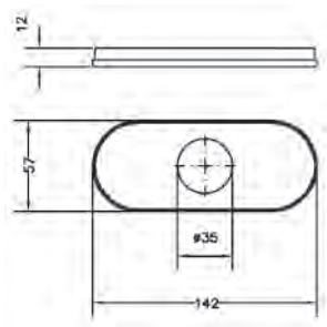
Ref.: P130 Placa adaptadora 4" 4" adaptor plate
