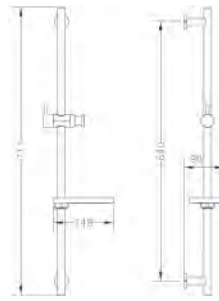
Ref.: 1639 45 Barra ducha metálica Metallic shower bar
