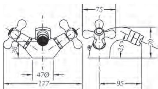
Ref.: 68515 09 45 66 Monobloc de bidé Bidet mixer
