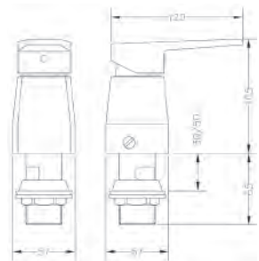
Ref.: 64142 16 45 66 Monomando de bidé con transmisión Single lever bidet mixer with diverter
