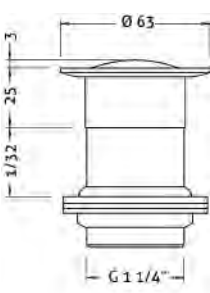
Ref.: 100207 45 Válvula click 1 1/4" 1 1/4" click valve
