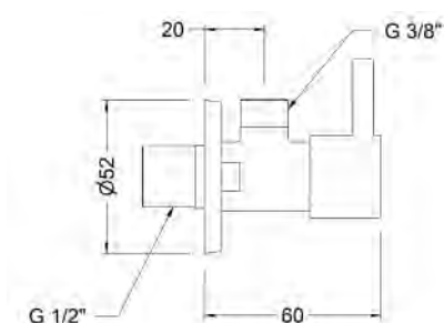
Ref.: 3104 04 Válvula de escuadra redonda 3/8" Round angle valve 3/8"
