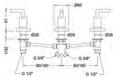
Ref.: 68113 12 45 66 Batería de baño con inversor Widespread bath mixer with diverter
