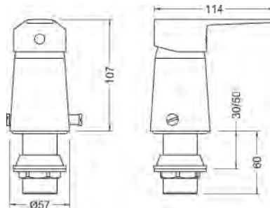
Ref.: 61142 28 45 66 Monomando de bidé con transmisión Single lever bidet mixer with diverter
