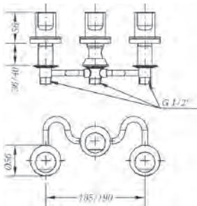
Ref.: 68142 07 45 66 Batería de bidé con transmisión Widespread bidet mixer with transmission Box: 1
