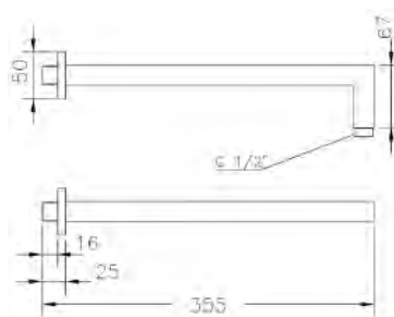
Ref.: B63113 26 Brazo pared cuadrado 35 cm Square wall arm 35 cm
