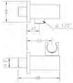
Ref.: 1649 04 Soporte ducha con toma cuadrado Square flexible wall conector
