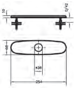
Ref.: P200 Placa adaptadora 8" 8" adaptor plate
