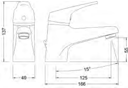
Ref.: 61130 22 45 66 Monomando de lavabo Plus Single lever Plus wash-basin mixer
