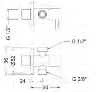
Ref.: 3107 03 Válvula de escuadra doble 1/2" - 3/8" ducha- inodoro Double angle valve 1/2" - 3/8" Box: 1 | Carton: 160 | Pallet: 3840
