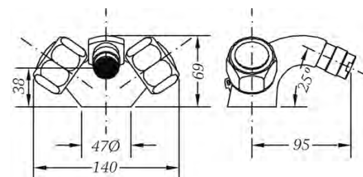
Ref.: 68140 11 45 66 Monobloc de bidé Bidet mixer
