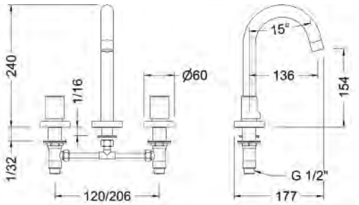
Ref.: 68124 07 45 66 Batería de lavabo caño cisne Widespread wash-basin mixer with swan pipe spout
