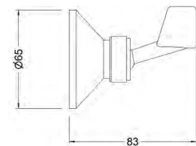
Ref.: 1647 45 Soporte ducha Clásico Classic shower holder
