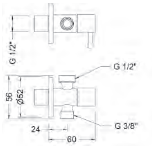
Ref.: 3108 03 Válvula de escuadra doble 1/2" - 3/8" Inox SS double angle valve 1/2" - 3/8" Box: 1 | Carton: 160 | Pallet: 3840
