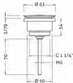
Ref.: 100205 45 Válvula click universal 1 1/4" 1 1/4" universal click valve
