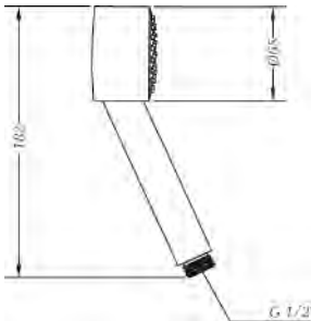
Ref.: 100197 45 00 Mango de ducha C1 jet C1 jet handshower
