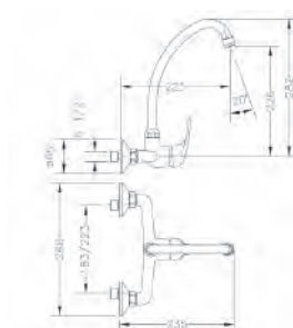
Ref.: 60194 05 45 66 Monomando de fregadera mural 8\"/>
