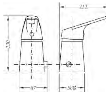
Ref.: 61142 22 45 66 Monomando de bidé con transmisión Single lever bidet mixer with diverter
