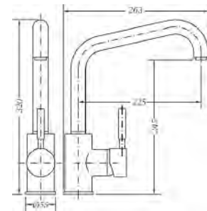
Ref.: 65204 18 45 66 Monomando de fregadera cartucho 40 Single lever sink mixer 40 cartridge
