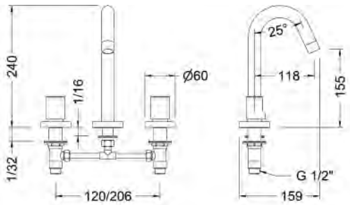
Ref.: 68125 07 45 66 Batería de lavabo caño inclinado Widespread wash-basin mixer with sloping pipe spout
