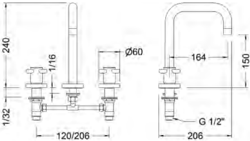
Ref.: 68120 08 45 66 Batería de lavabo caño recto Widespread wash-basin mixer with straight pipe spout
