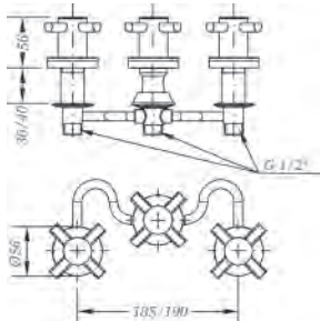
Ref.: 68142 08 45 66 Batería de bidé con transmisión Widespread bidet mixer with transmission
