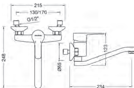
Ref.: 61196 28 45 66 Monomando de fregadera caño inferior elevado Wall single lever sink mixer low spout
