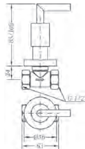
Ref.: 68170 12 45 66 Llave de paso 1/2\"/> Stopcock 1/2\" Box: 1
