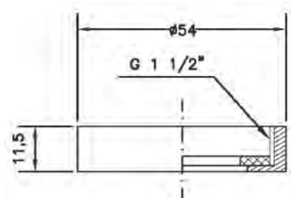
Ref.: 100134 08 Tuerca para sifon 1 1/2" 1 1/2" siphon nut
