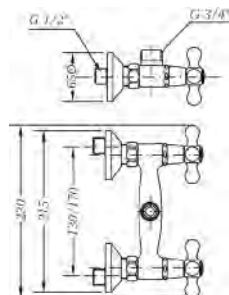
Ref.: 568555 45 Cuerpo grupo mural 15 cm Wall body mixer 15 cm
