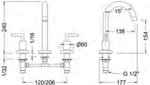
Ref.: 68124 12 45 66 Batería de lavabo caño cisne Widespread wash-basin mixer with swan pipe spout Box: 1
