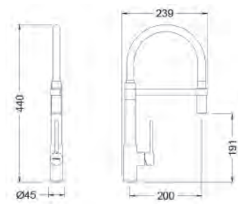
Ref.: 65219 18 45 66 Monomando de fregadera cartucho 25 apertura en frío Single lever sink mixer 25 cartridge cold start Box: 1 | Carton: 4 | Pallet: 48
