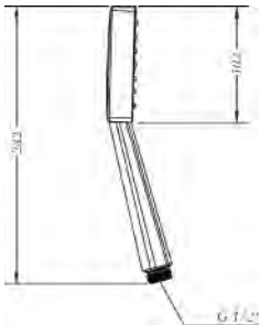
Ref.: DXK1 45 Mango de ducha K1 jets K1 jet handshower
