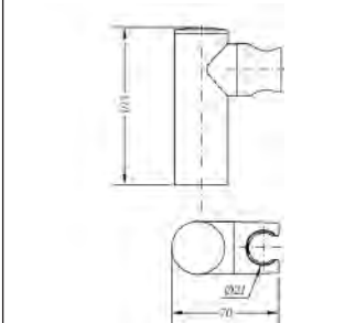
Ref.: 100153 45 Soporte ducha cilíndrico Cylindrical shower holder
