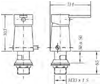
Ref.: 65142 29 45 66 Monomando de bidé con transmisión Single lever bidet mixer with diverter
