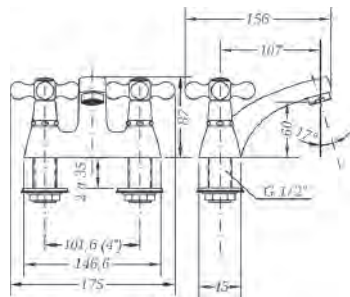
Ref.: 68511 09 45 66 Mezclador lavabo 4" Wash-basin mixer 4"
