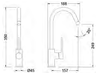
Ref.: 65403 18 45 66 Monomando de fregadera cartucho 25 apertura en frío Single lever sink mixer 25 cartridge cold start
