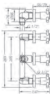
Ref.: 68116 08 45 66 Grupo ducha empotrado 8" con inversor Built-in 8" bath mixer with diverter Box: 1
