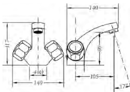
Ref.: 68130 11 45 66 Monobloc de lavabo Wash-basin mixer
