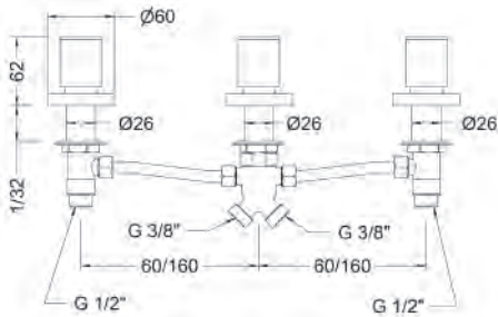
Ref.: 68113 07 45 66 Batería de baño con inversor Widespread bath mixer with diverter
