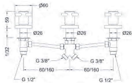
Ref.: 68113 08 45 66 Batería de baño con inversor Widespread bath mixer with diverter
