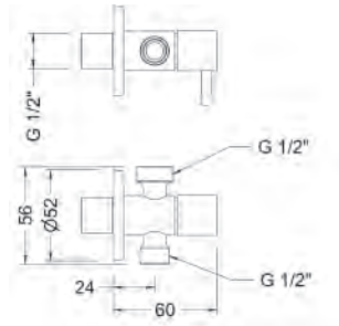
Ref.: 3107 04 Válvula de escuadra doble 1/2" - 1/2" ducha- inodoro Double angle valve 1/2" - 1/2" Box: 1 | Carton: 160 | Pallet: 3840
