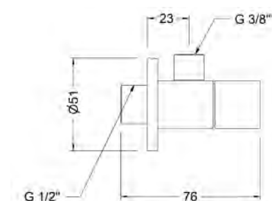
Ref.: 3106 04 Válvula de escuadra cuadrada 3/8" Square angle valve 3/8"
