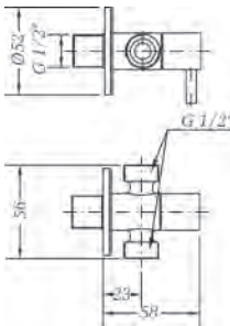
Ref.: 3108 04 Válvula de escuadra doble 1/2" - 1/2" Inox SS double angle valve 1/2" - 1/2" Box: 1 | Carton: 160 | Pallet: 3840
