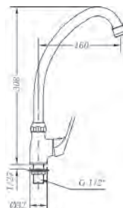
Ref.: 1009 04 Grifo fregadera 1 agua cartucho 25 One-water sink tap 25 cartridge
