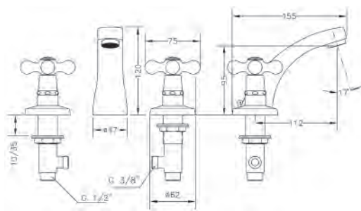
Ref.: 68510 09 45 66 Batería lavabo Widespread wash-basin mixer
