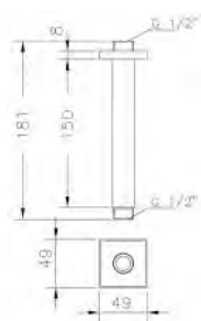
Ref.: 1672 45 Brazo a techo cuadrado 15 cm Square roof arm 15 cm
