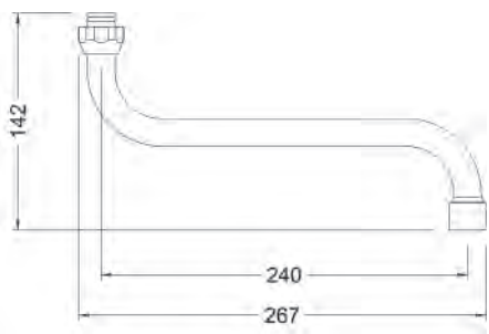
Ref.: 68904 45 Caño bajo tubo 24 cm Low tube spout 24 cm
