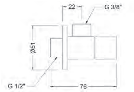
Ref.: 3106 05 Válvula de escuadra cuadrada 1/2" Square angle valve 1/2" Box: 2 | Carton: 120 | Pallet: 4320
