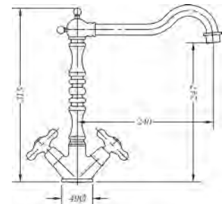
Ref.: 68595 09 43 66 Monobloc de fregadera bronce Bronze sink mixer
