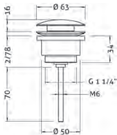
Ref.: 100211 43 Válvula click "Luxe" bronce 1 1/4" 1 1/4" "Luxe" click valve bronze
