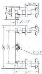
Ref.: 68115 08 45 66 Grupo ducha empotrado 8\"/> Built-in 8" shower mixer Box: 1
