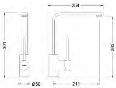
Ref.: 65404 18 45 66 Monomando de fregadera cartucho 35 apertura en frío Single lever sink mixer 35 cartridge cold start
