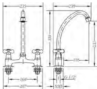
Ref.: 68194 09 45 66 Mezclador mesada 6" caño tubo 6" deck mixer with swan neck spout
