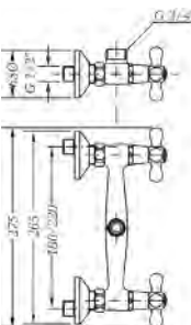
Ref.: 568565 45 Cuerpo grupo mural 20 cm Wall body mixer 20 cm
