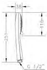
Ref.: DXO3 45 Mango de ducha O3 jets O3 jets handshower
