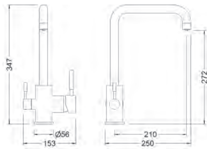
Ref.: 65702 18 45 66 Monomando de fregadera 3 vías Single lever 3-way sink mixer Box: 1 | Carton: 4 | Pallet: 96
