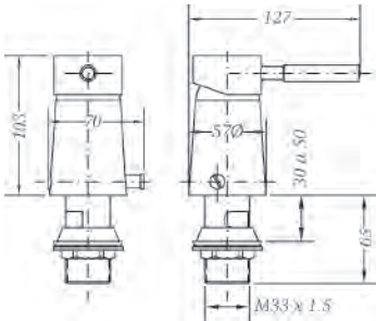
Ref.: 65142 18 45 66 Monomando de bidé con transmisión Single lever bidet mixer with diverter
