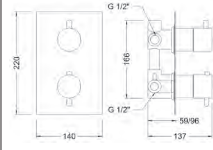
Ref.: 64111 14 45 67 Termostática empotrada 3 vías Built-in 3-way thermostatic
