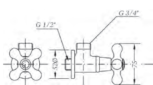
Ref.: 568575 45 Cuerpo grifo mural Wall body tap
