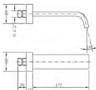
Ref.: 1674 45 Caño mural baño cuadrado Square wall bath spout
