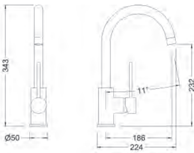
Ref.: FRT65402 Monomando de fregadera cartucho 35 apertura en frío Single lever sink mixer 35 cartridge cold start Box: 1 | Carton: 8 | Pallet: 96
