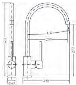
Ref.: FRT65401 Monomando de fregadera cartucho 25 apertura en frío Single lever sink mixer 25 cartridge cold start Box: 1 | Carton: 8 | Pallet: 96
