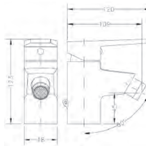
Ref.: 64140 16 45 66 Monomando de bidé Single lever bidet mixer
