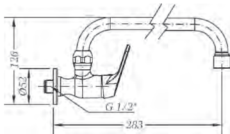
Ref.: 1008 04 Grifo mural con tubo 24 cm 1 agua cartucho 25 One-water wall sink tap spout 24 cm 25 cartridge
