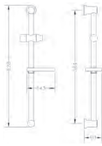
Ref.: 1638 45 Barra ducha redonda Round shower bar
