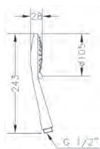
Ref.: DXT3 45 Mango de ducha T3 jets T3 jets handshower Box: 1 | Carton: 36 | Pallet: 324
