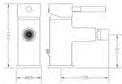
Ref.: 65145 18 45 66 Monomando de bidé Single lever bidet mixer
