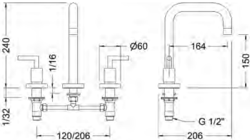
Ref.: 68120 12 45 66 Batería de lavabo caño recto Widespread wash-basin mixer with straight pipe spout Box: 1
