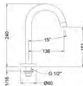
Ref.: 68916 45 Caño encimera cisne tubo Swan neck pipe spout
