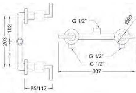
Ref.: 68115 12 45 66 Grupo ducha empotrado 8\"/> Built-in 8\" shower mixer Box: 1
