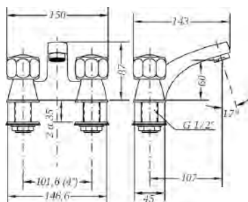
Ref.: 68122 11 45 66 Mezclador lavabo 4" Wash-basin mixer 4"
