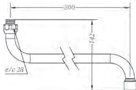
Ref.: 68909 45 Caño bajo tubo 30 cm Low tube spout 30 cm
