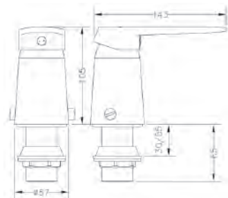
Ref.: 62142 31 45 66 Monomando de bidé con transmisión Single lever bidet mixer with diverter
