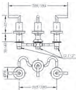
Ref.: 68142 12 45 66 Batería de bidé con transmisión Widespread bidet mixer with transmission Box: 1
