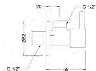
Ref.: 3104 05 Válvula de escuadra redonda 1/2" Round angle valve 1/2"
