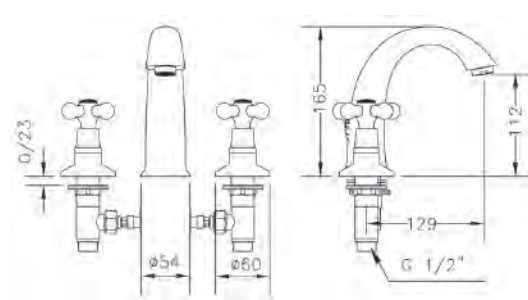
Ref.: 68120 09 45 66 Batería lavabo Widespread wash-basin mixer
