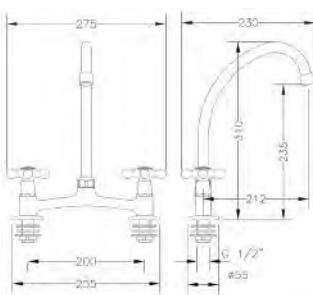
Ref.: 68545 09 45 66 Mezclador mesada 8" caño tubo 8" deck mixer with swan neck spout
