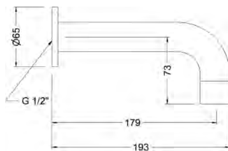
Ref.: 1668 45 Caño mural baño cilíndrico Round wall bath spout
