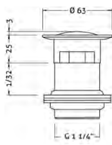
Ref.: 100206 45 Válvula click 1 1/4" con rebodadero 1 1/4" click valve with overflow
