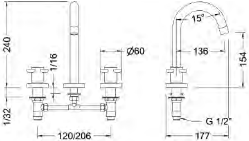
Ref.: 68124 08 45 66 Batería de lavabo caño cisne Widespread wash-basin mixer with swan pipe spout
