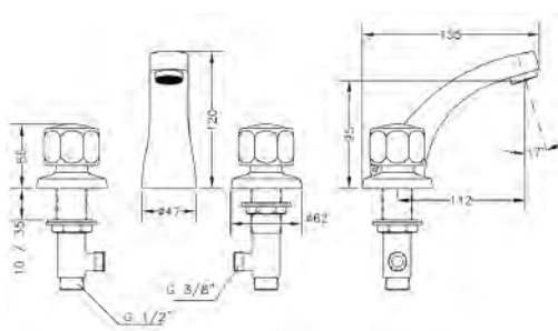
Ref.: 68120 11 45 66 Batería de lavabo Widespread wash-basin mixer
