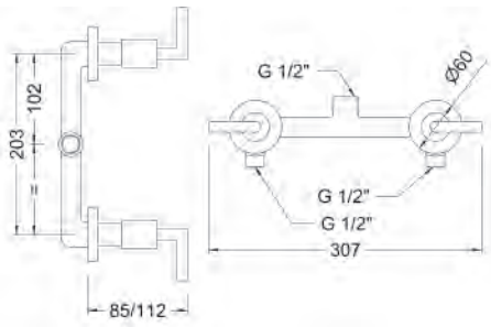
Ref.: 68115 07 45 66 Grupo ducha empotrado 8" Built-in 8" shower mixer Box: 1
