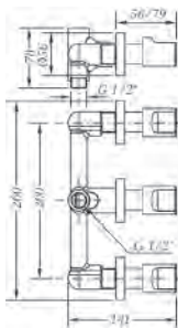
Ref.: 68116 07 45 66 Grupo baño empotrado 8" con inversor Built-in 8" bath mixer with diverter Box: 1
