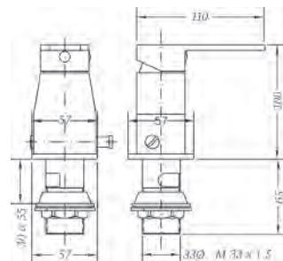
Ref.: 63142 26 45 66 Monomando de bidé con transmisión Single lever bidet mixer with diverter
