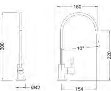
Ref.: 65700 18 45 66 Grifo de 1 vía One way tap Box: 80 | Carton: 960 | Pallet: 7680
