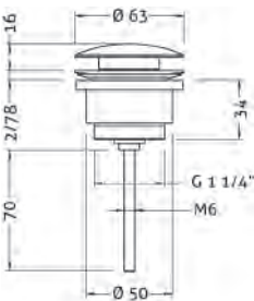
Ref.: 100211 45 Válvula click "Luxe" 1 1/4" 1 1/4" "Luxe" click valve
