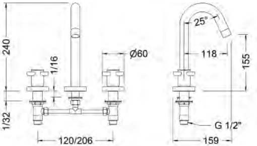
Ref.: 68125 08 45 66 Batería de lavabo caño inclinado Widespread wash-basin mixer with sloping pipe spout
