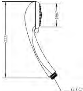
Ref.: DXE2 45 Mango de ducha E2 jets E2 jets handshower
