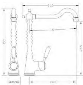
Ref.: 68201 39 45 66 Monomando de fregadera cromo Chromed sink mixer
