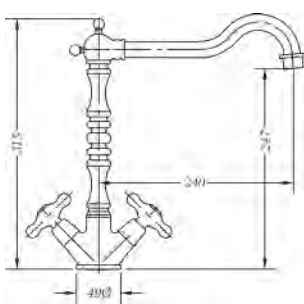
Ref.: 68595 09 45 66 Monobloc de fregadera cromo Chromed sink mixer
