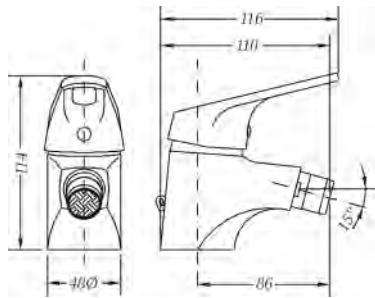
Ref.: 60140 22 45 66 Monomando de bidé Single lever bidet mixer
