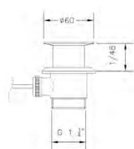
Ref.: 100203 45 Válvula automática metálica 1 1/4" 1 1/4" metallic automatic valve
