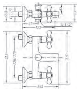
Ref.: 68525 09 45 66 Mezclador de baño con kit Bath mixer with kit
