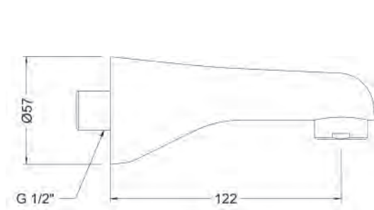
Ref.: 1667 45 Caño mural baño fundido Casted wall bath spout Box: 1 | Carton: 60 | Pallet: 1080
