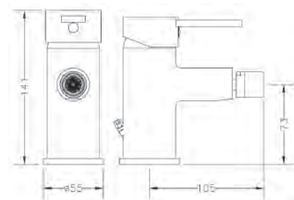
Ref.: 65145 29 45 66 Monomando de bidé Single lever bidet mixer
