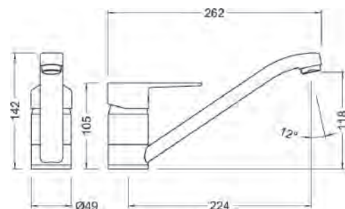
Ref.: 61200 28 45 66 Monomando de fregadera Single lever sink mixer
