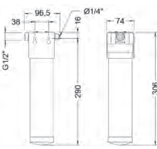
Ref.: FT00 Kit declorador Filtro declorador Box: 80 | Carton: 960 | Pallet: 7680
