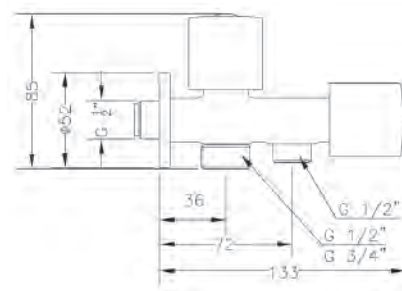
Ref.: 1023 04 Grifo doble combinable 1/2\"/>
