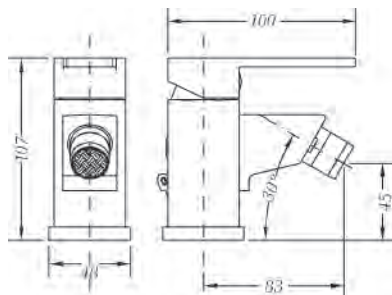
Ref.: 63140 26 45 66 Monomando de bidé Single lever bidet mixer
