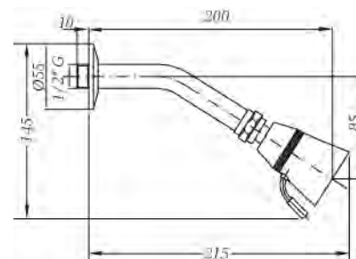
Ref.: 1698 45 Rociador ducha con brazo Wall shower arm and spray
