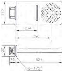
Ref.: 1643 45 Rociador doble función cascada-lluvia Shower head double function waterfall-rain Box: 1 | Carton: 2 | Pallet: 12
