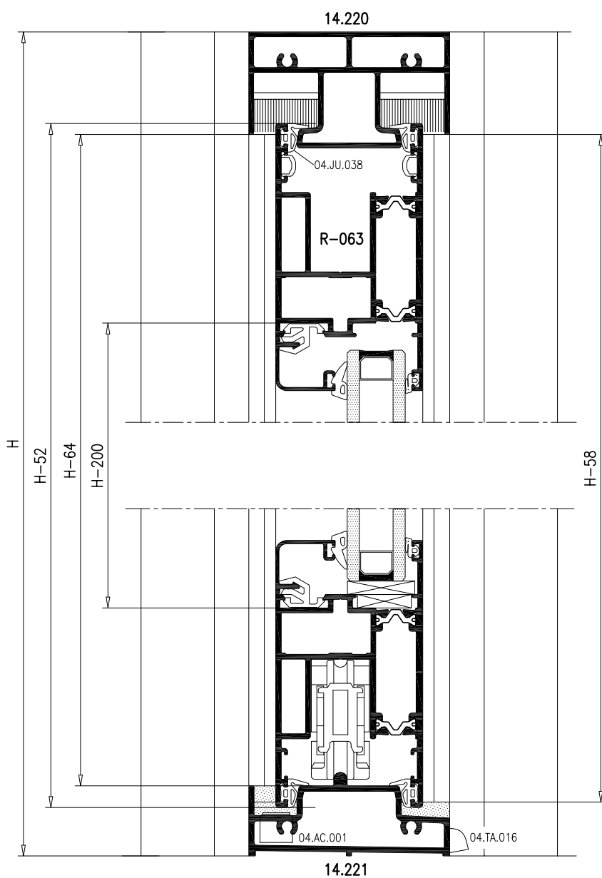
SECCION A-A'
