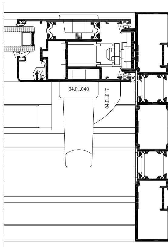
SECCION A-A'
