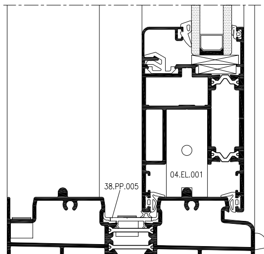
SECCION B-B'
