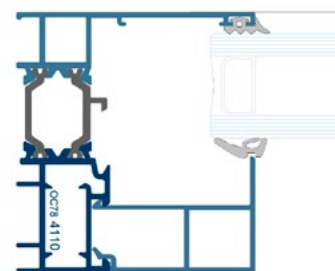
SECCIÓN LATERAL MARCO FIJO
