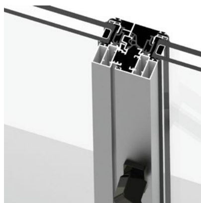
Central asimétrico desde el interior
