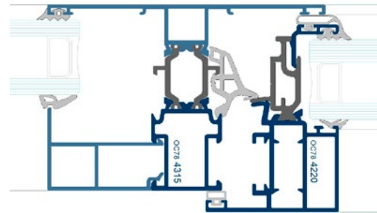
SECCIÓN CENTRAL
