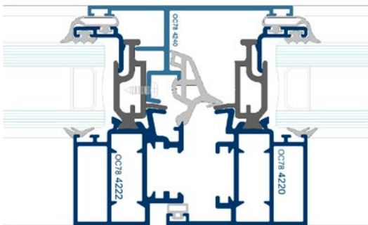
SECCIÓN NUDO CENTRAL
