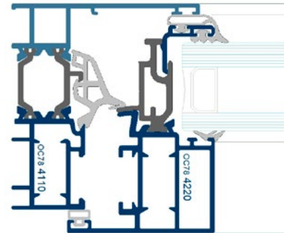
SECCIÓN LATERAL
