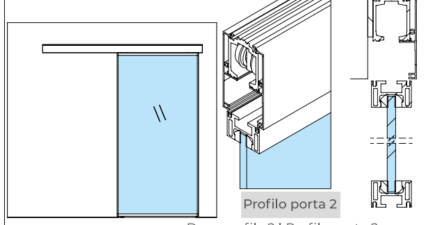
Door profile 2 | Perfil puerta 2
