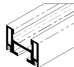
Traversa per profilo a sbalzo Traverse for offset door profile Travesaño para perfil con eje desplazado
