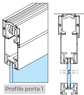
Door profile 1 | Perfil puerta 1
