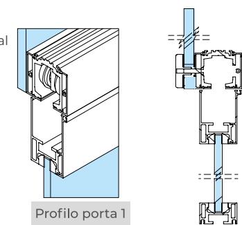
Door profile 1 | Perfil puerta 1
