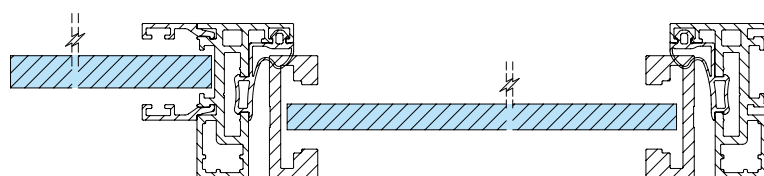
SEZIONE B-B SCALA 1:1
