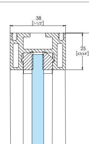
Door profile 1 | Perfil puerta 1
