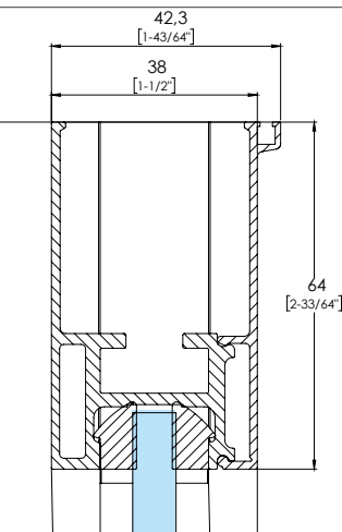
Door profile 2 | Perfil puerta 2
