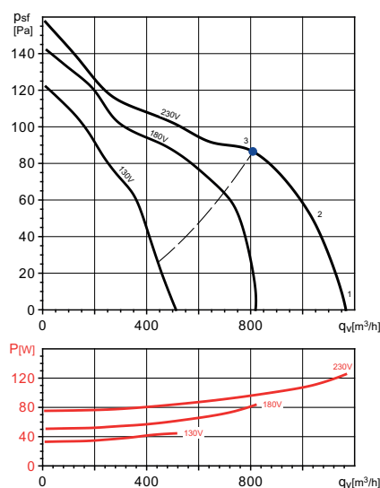
CQ /6 7/7 72W
