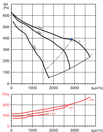
CQ /4 10/10 550W
