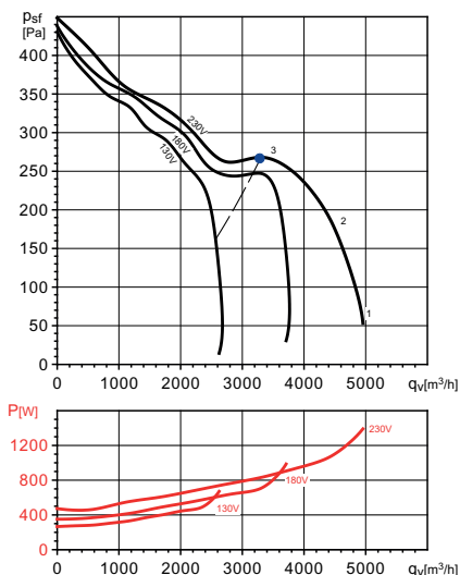
CQ /6 12/12 736W
