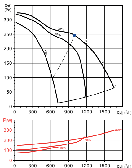
CQ /4 7/7 147W
