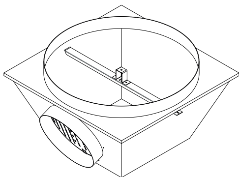
Plenum + acoplamientos montados (Excepto para Ø 600 mm)
