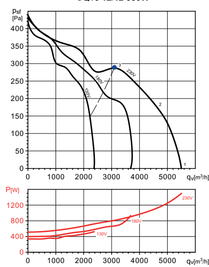
CQ /6 12/12 550W
