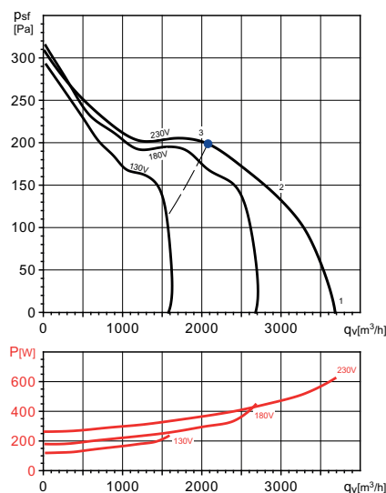
CQ /6 10/10 245W
