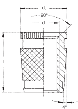
Tipo 0932
