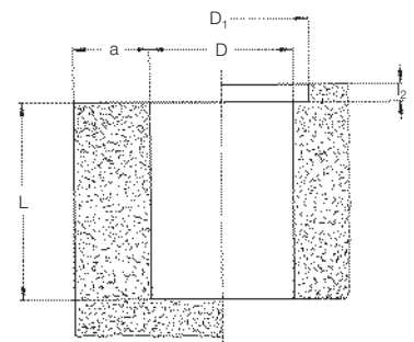
Dimensiones del alojamiento ①
