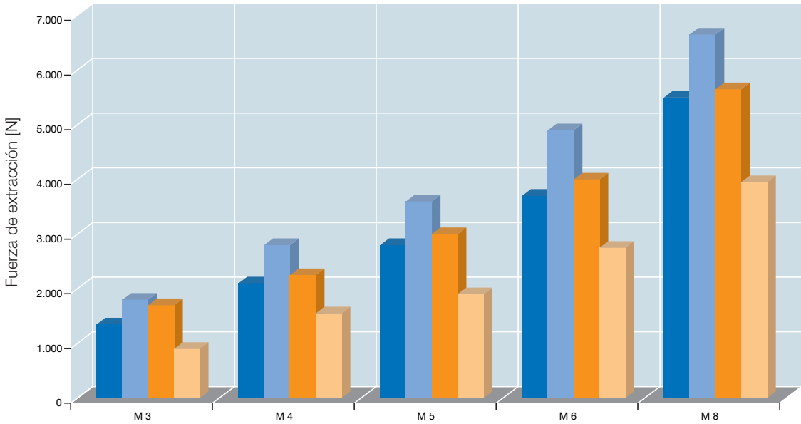
Valores de extracción HITSERT® M 3 a M 8
