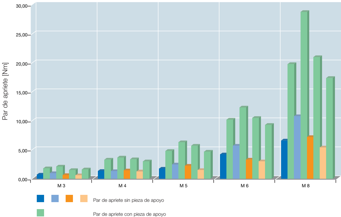
Pares de apriete SPREDSERT® 1 + 2 / M 3 a M 8
