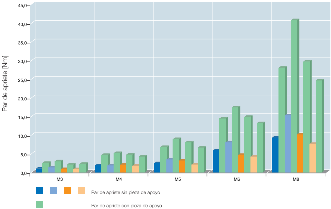
Pares de apriete SONICSERT® M 3 a M 8
