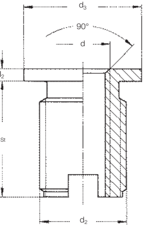
Dimensiones de alojamiento recomendadas -D- para QUICKSERT® en diferentes materiales ®
