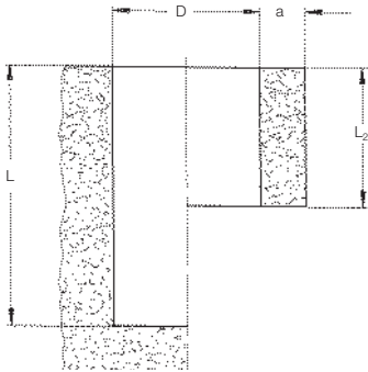
Dimensiones del alojamiento ①
