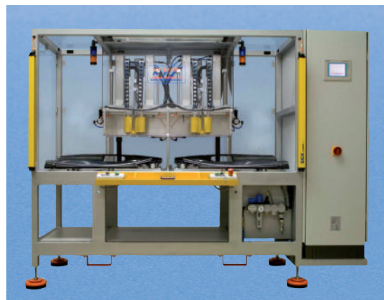
Máquina de colocación por calor con diseño especial para integración simultánea de 6 insertos en dos puertas de automóvil.
