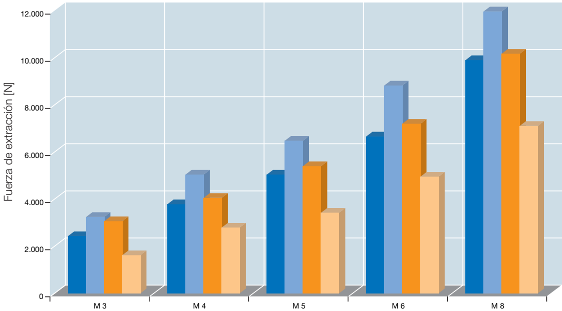
Valores de extracción QUICKSERT® M 3 a M 8
