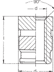
Tipo 0733
