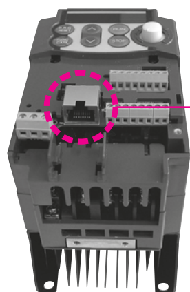
Puerto de comunicación RS-485
