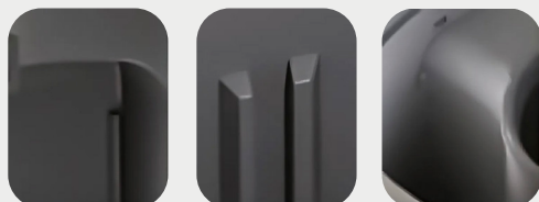
Guías verticales para el montaje del tabique sifónico en la arqueta.
