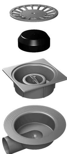
Caldereta sifónica salida horizontal
