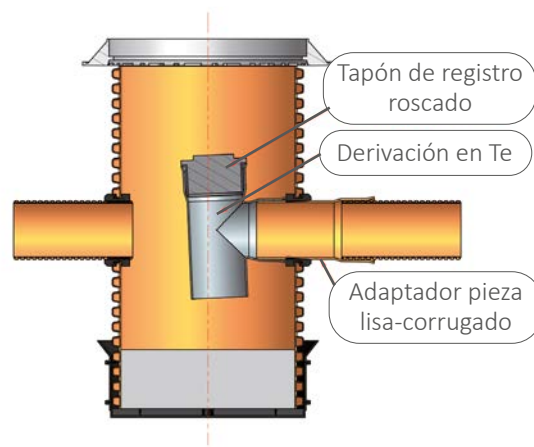
Arqueta sifónica
