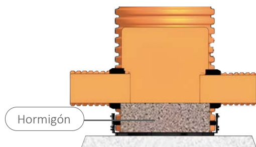
Acabado del fondo del pozo con base estanca (necesario con freático)
