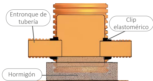
Acabado del fondo del pozo rematado con hormigón (solamente recomendable sin freático)
