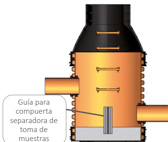
Pozo tomamuestras
