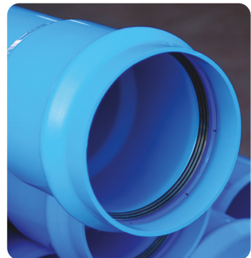
Le joint à bague autobloquante assure l'étanchéité parfaite des assemblages.
