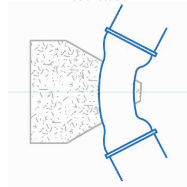
Anclajes en cambios de dirección
