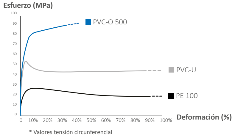
Curvas de esfuerzo-deformación
