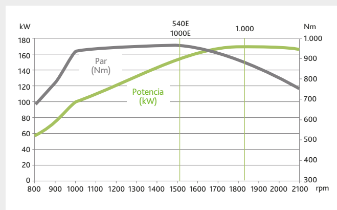
↑ Concepto de bajo régimen del motor con curvas de potencia y par optimizadas. (6230 TTV y 6230 TTV HD - curva del motor de 230 CV mostrada en el gráfico).
